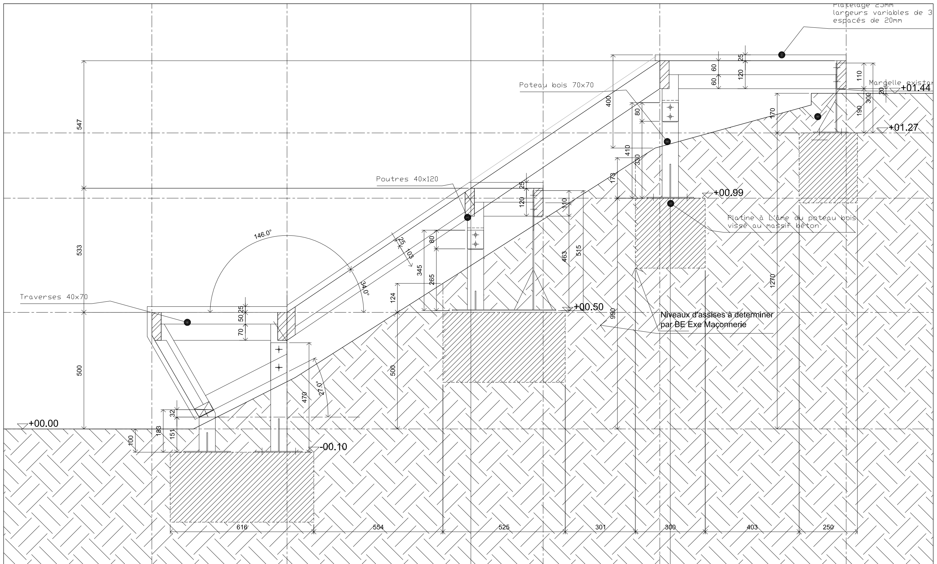
COUPE TRANSVERSALE SUR L'UNITE 01 - MODIFICATION DE L'ALTIMETRIE DU TALUS Structure - Entraxes 40cm - (niv. relevé du maçon du 09/11/21)
