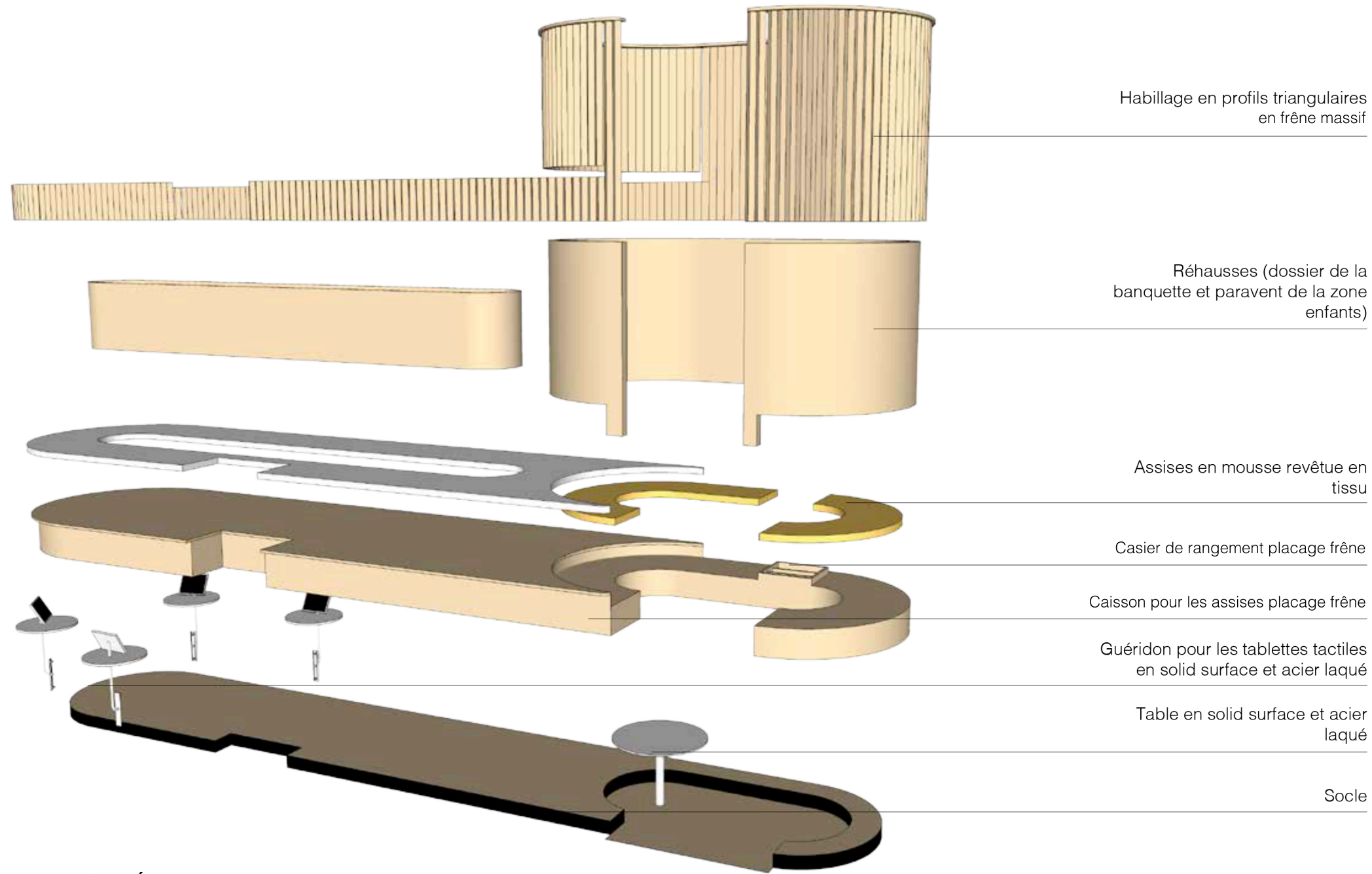
VUE EN ECLATÉE
