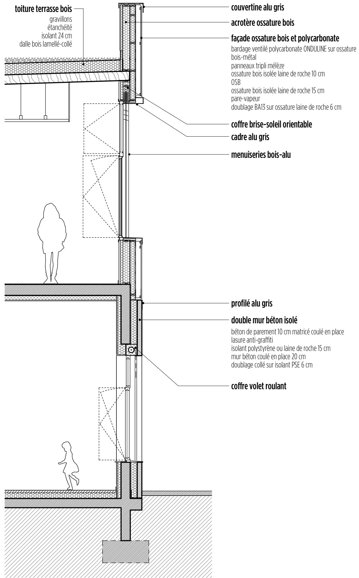
coupe façade Nord
