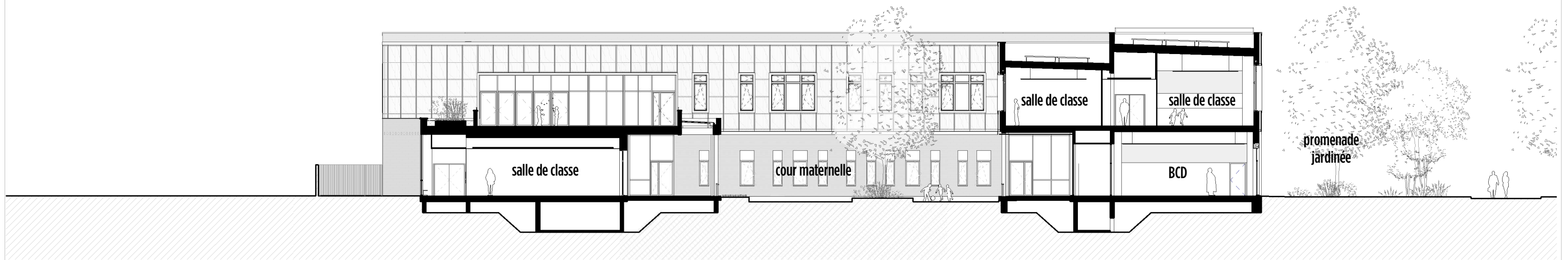
coupe CC
