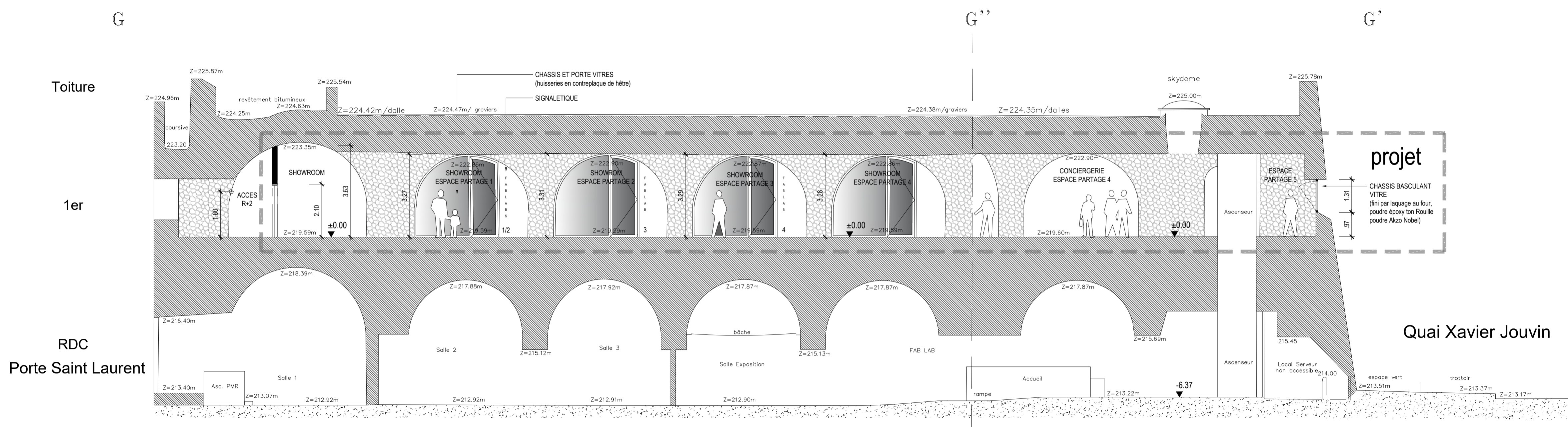
COUPE GG'
