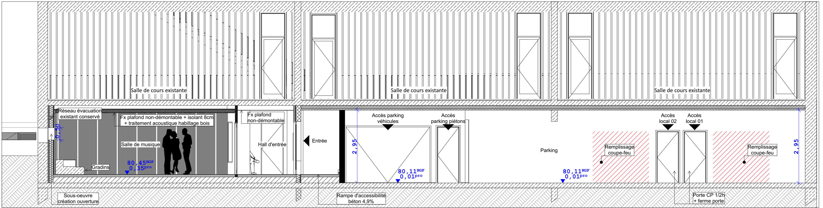
Coupe DD projeté
