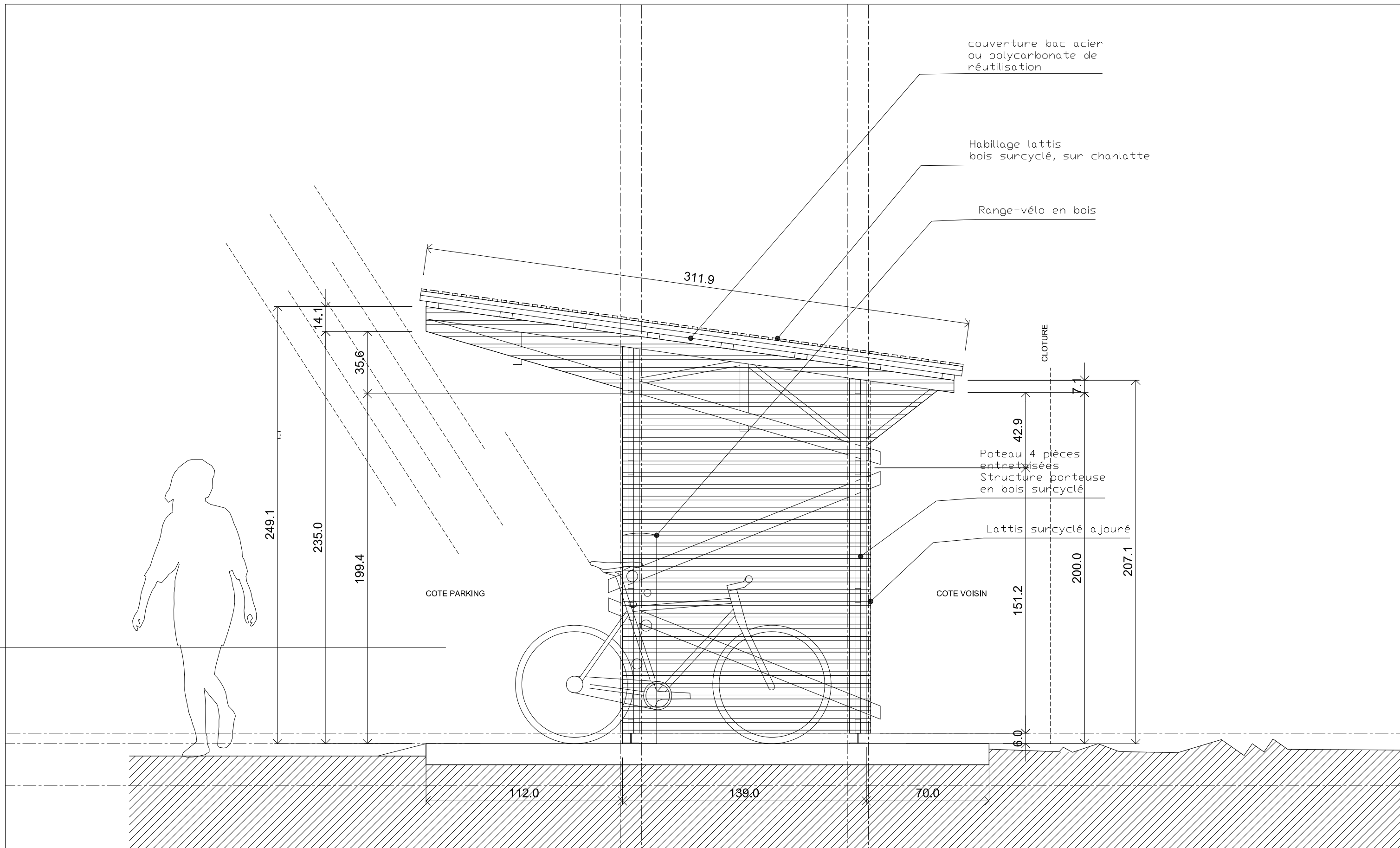
VUE DE DROITE Dimensions, nomenclatures
