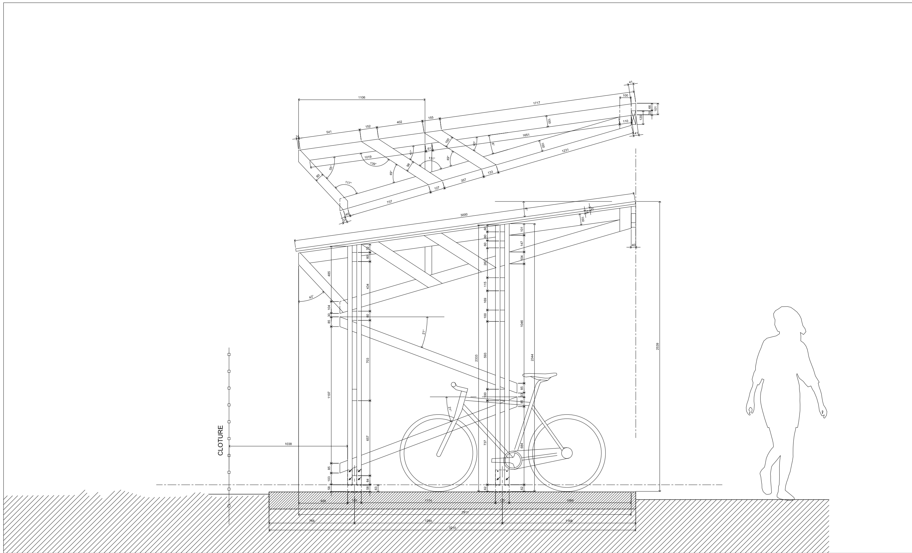
PORTIQUE (CENTRAL) Elevation
