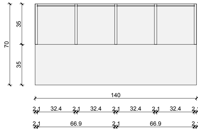
Plan en vue de dessus
