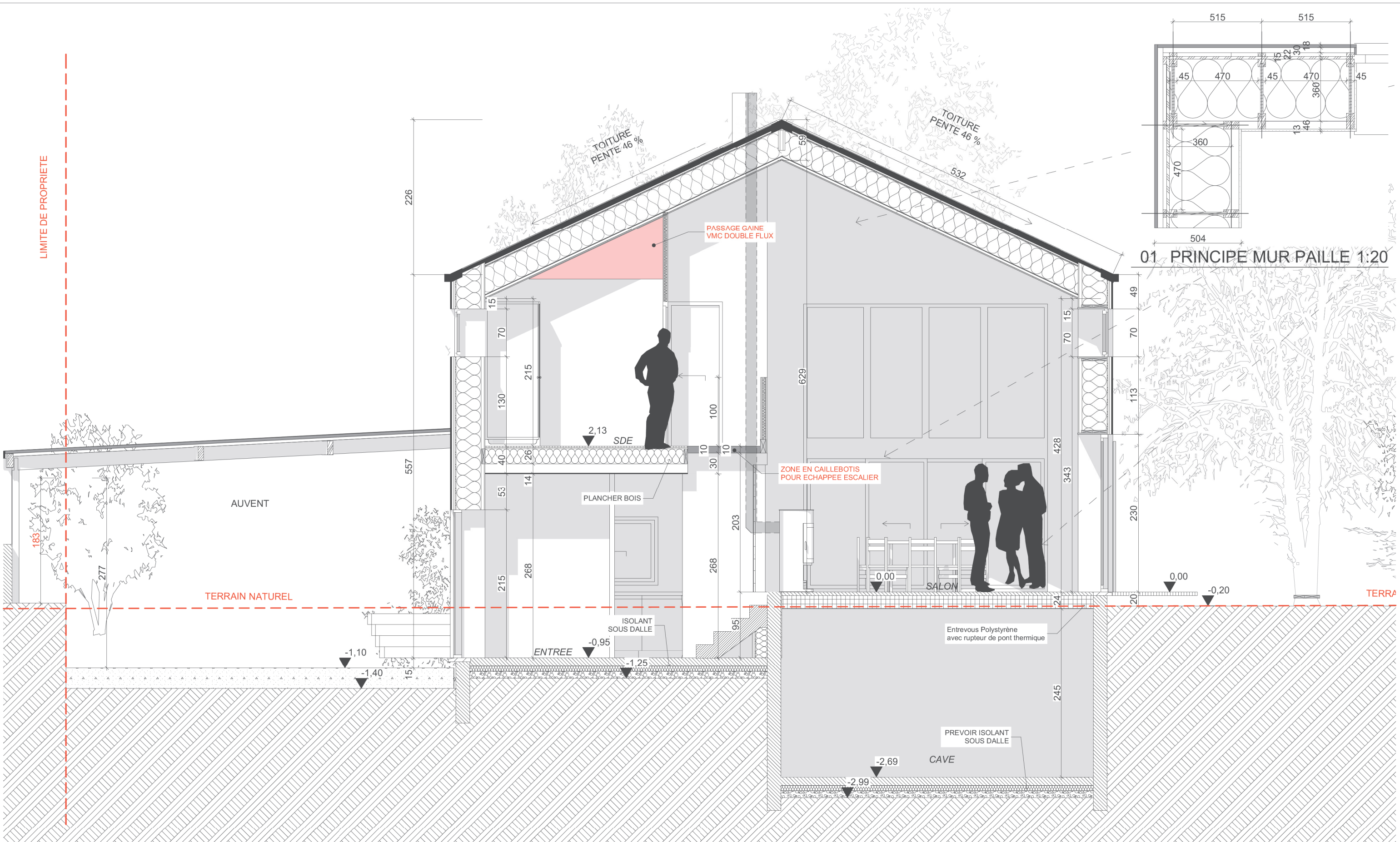
COUPE A
