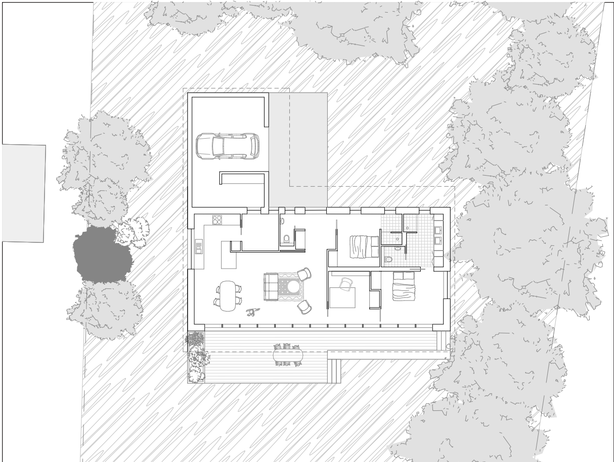
Plan RDC 1 300 ⓪
