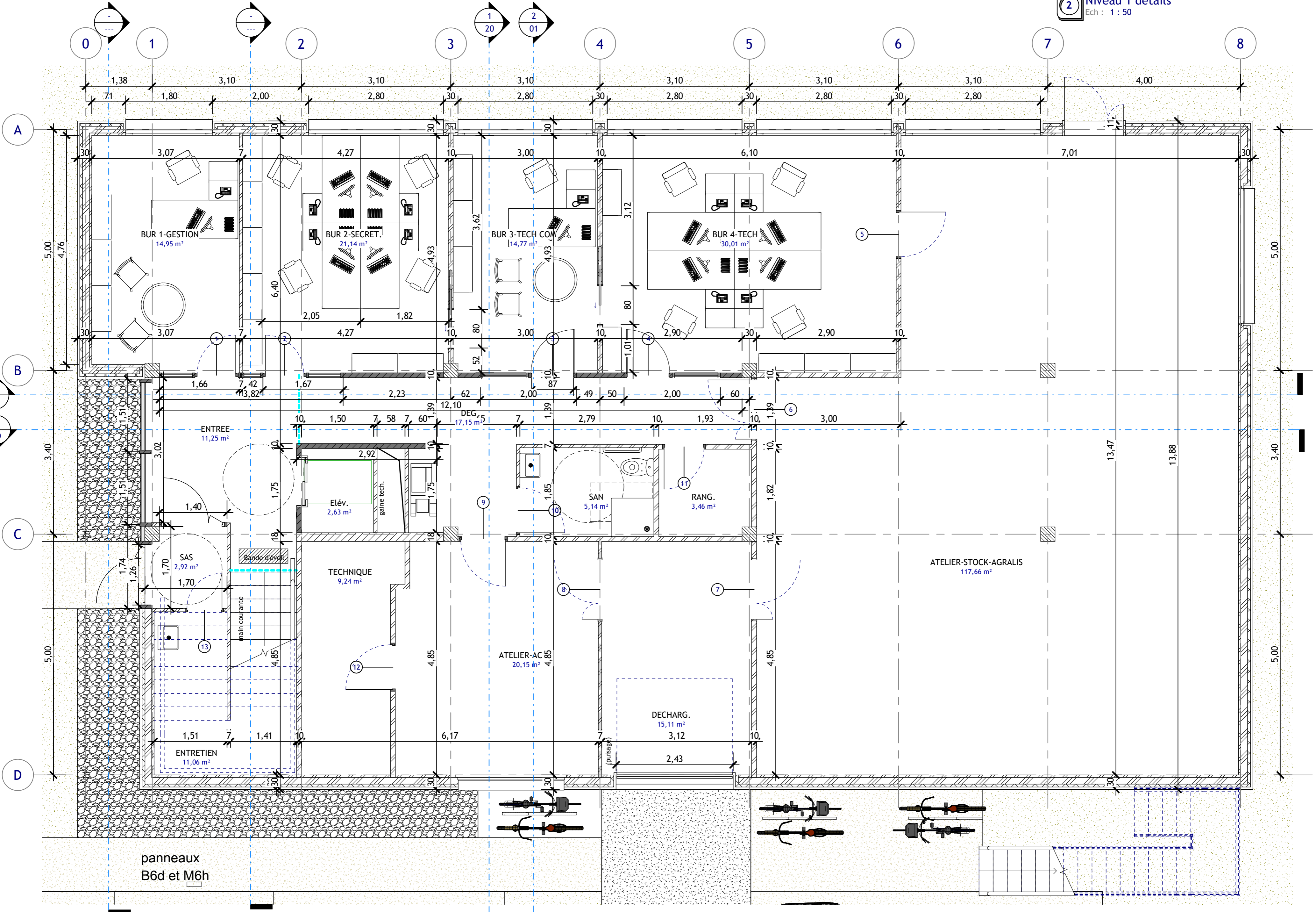
1 Niveau 0 détails Ech : 1 : 50
