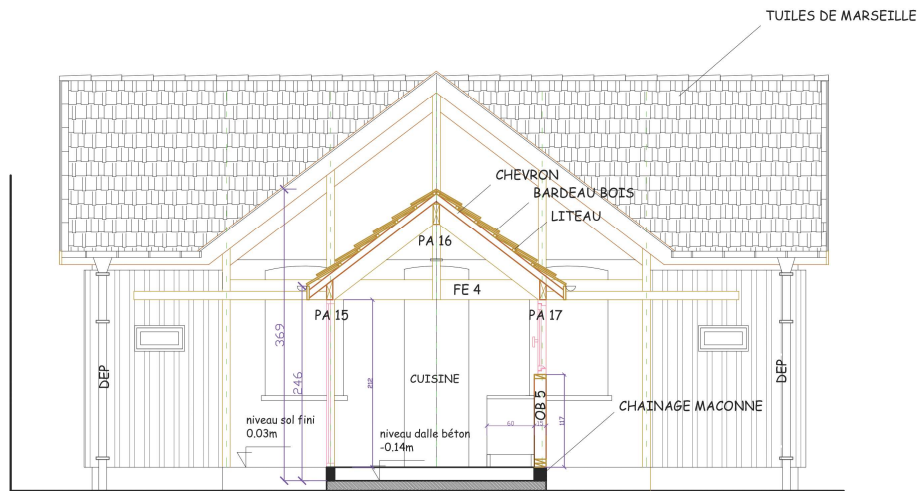
COUPE 6
