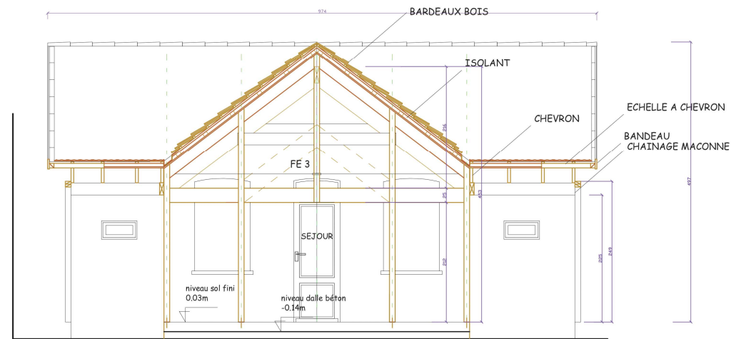
COUPE 5
