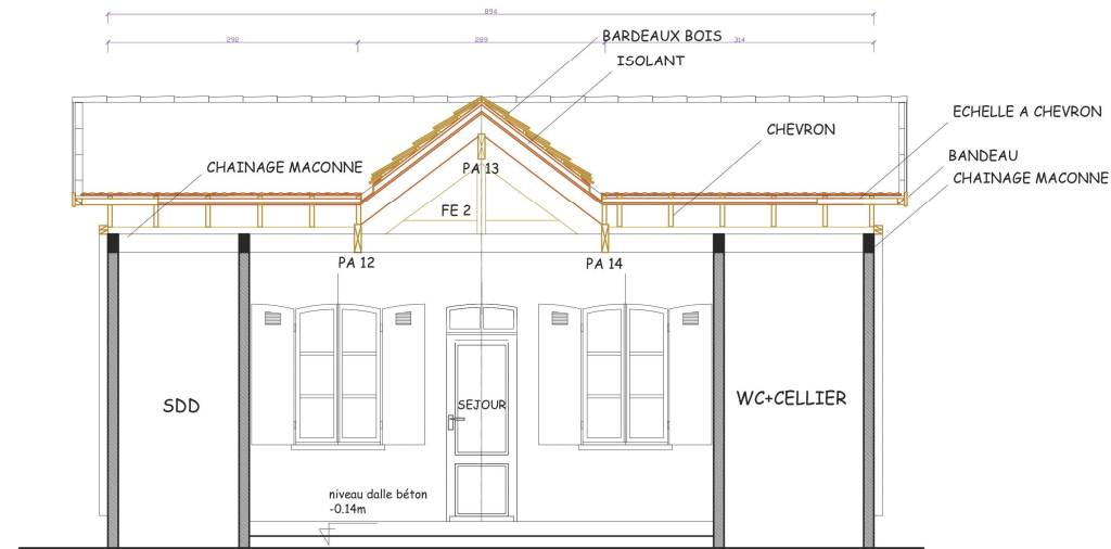
COUPE 4
