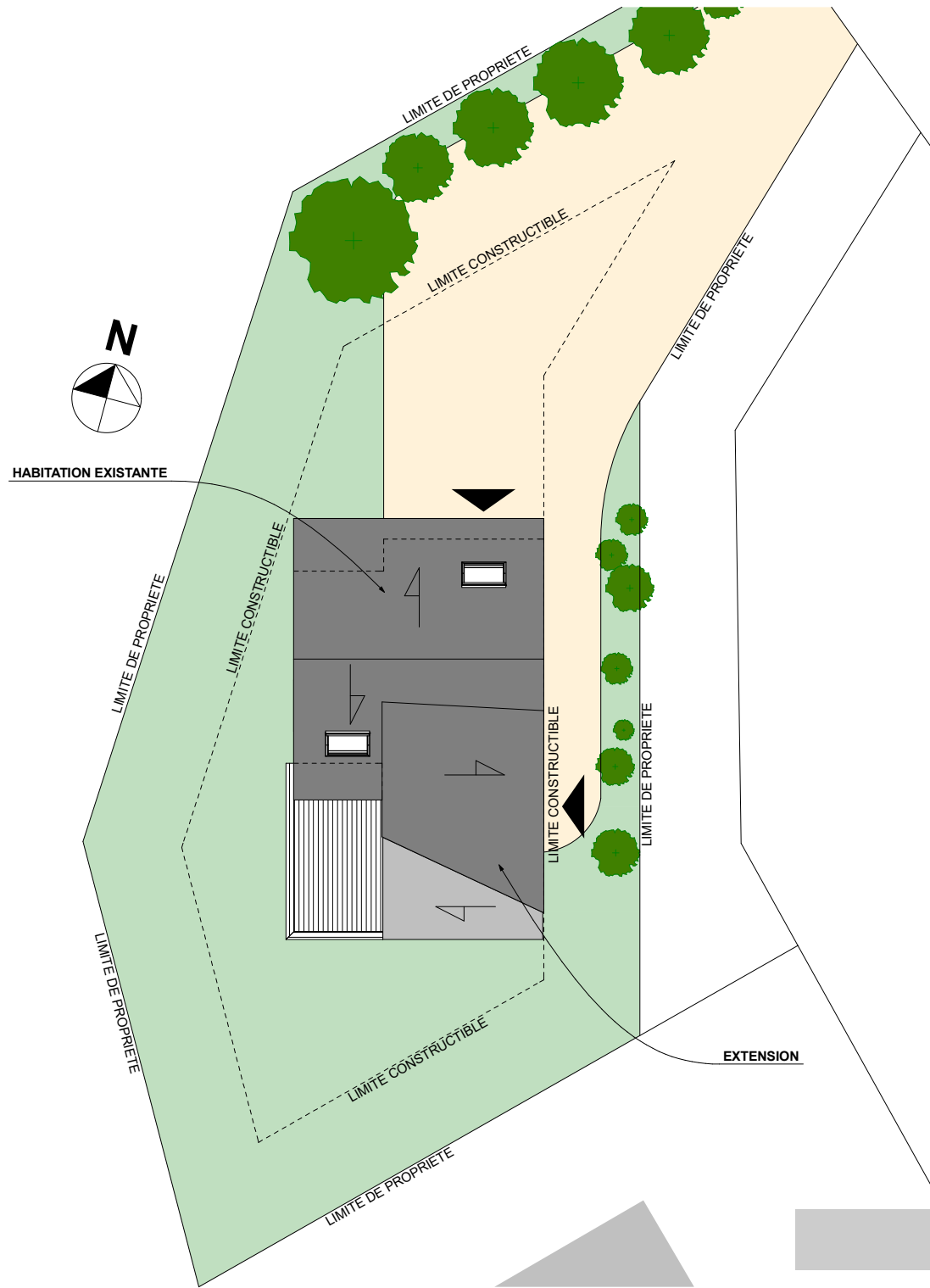
PLAN DE MASSE EXTENSION FP - GUILLAUME RÉTIF
