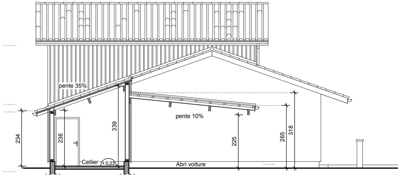
COUPE AA (log.t 5)
