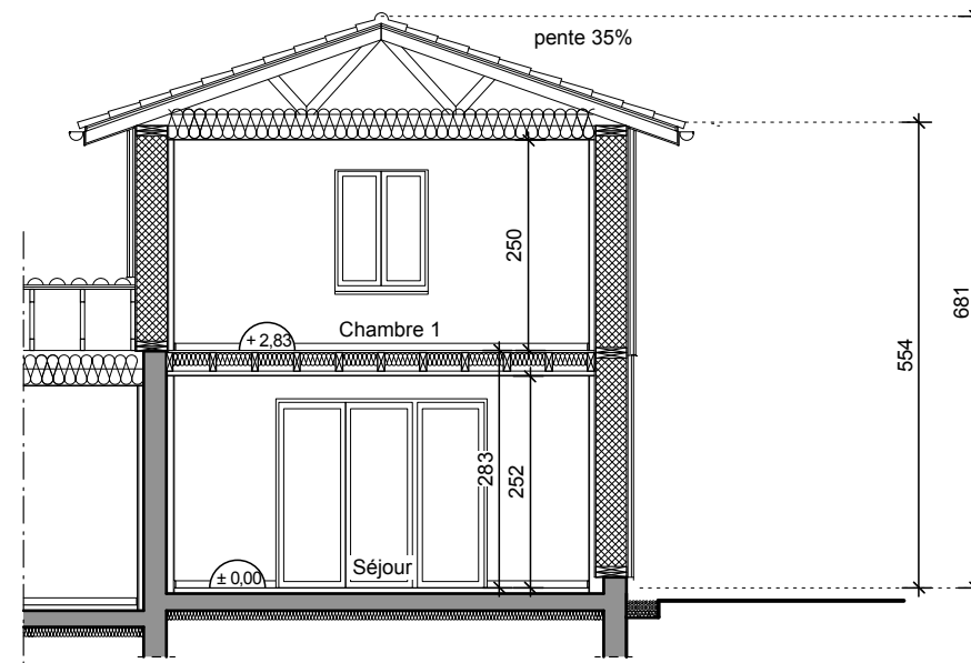
COUPE CC (log.t 14)
