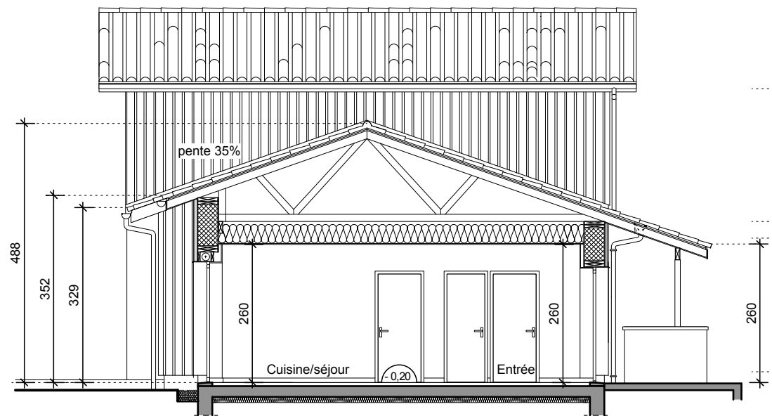
COUPE AA (log.t 12)
