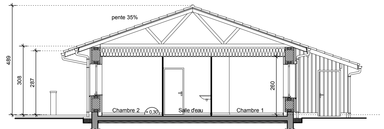
COUPE BB (log.t 5)
