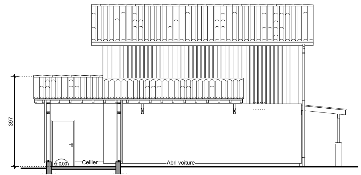
COUPE BB (log.t 8)
