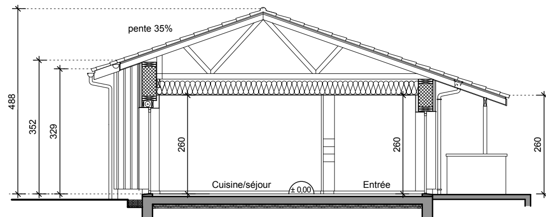
COUPE BB (log.t 10)
