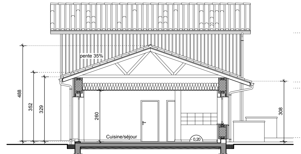
COUPE BB (log.t 13)
