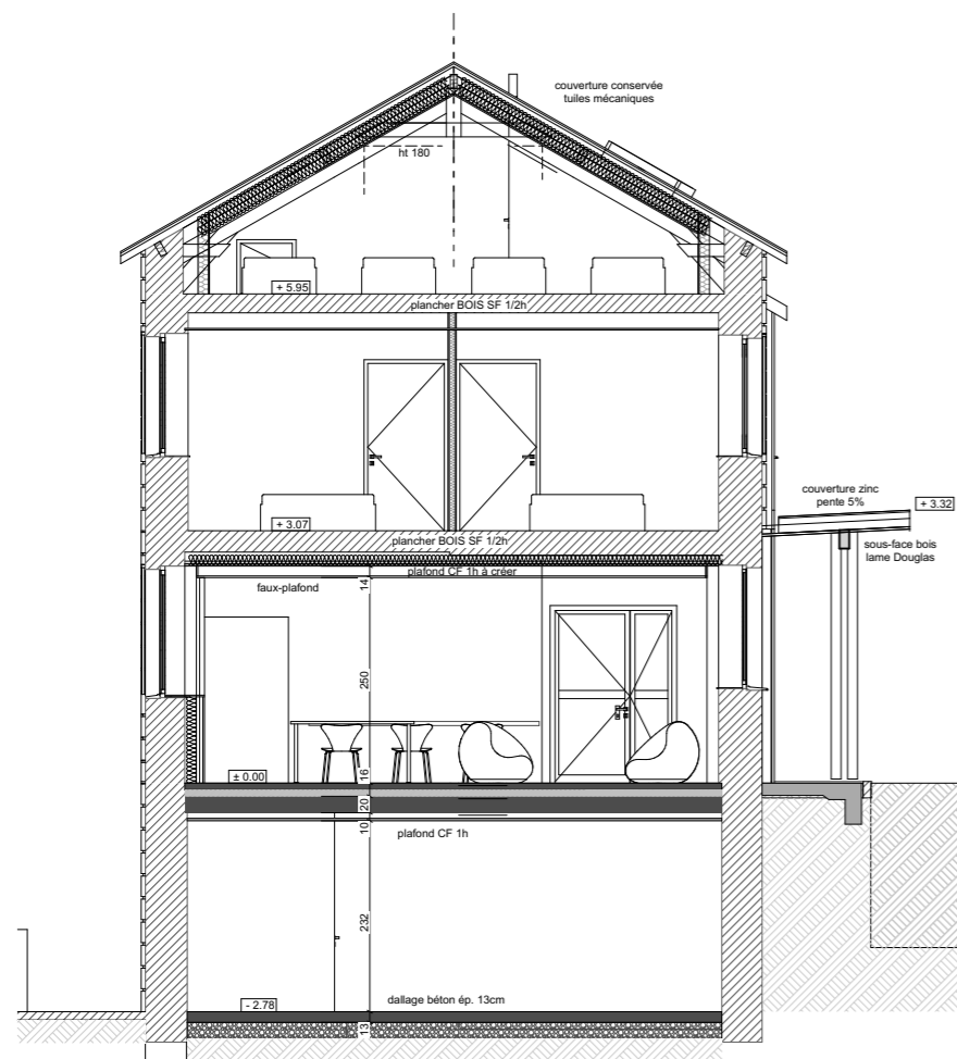
Coupe A-A
