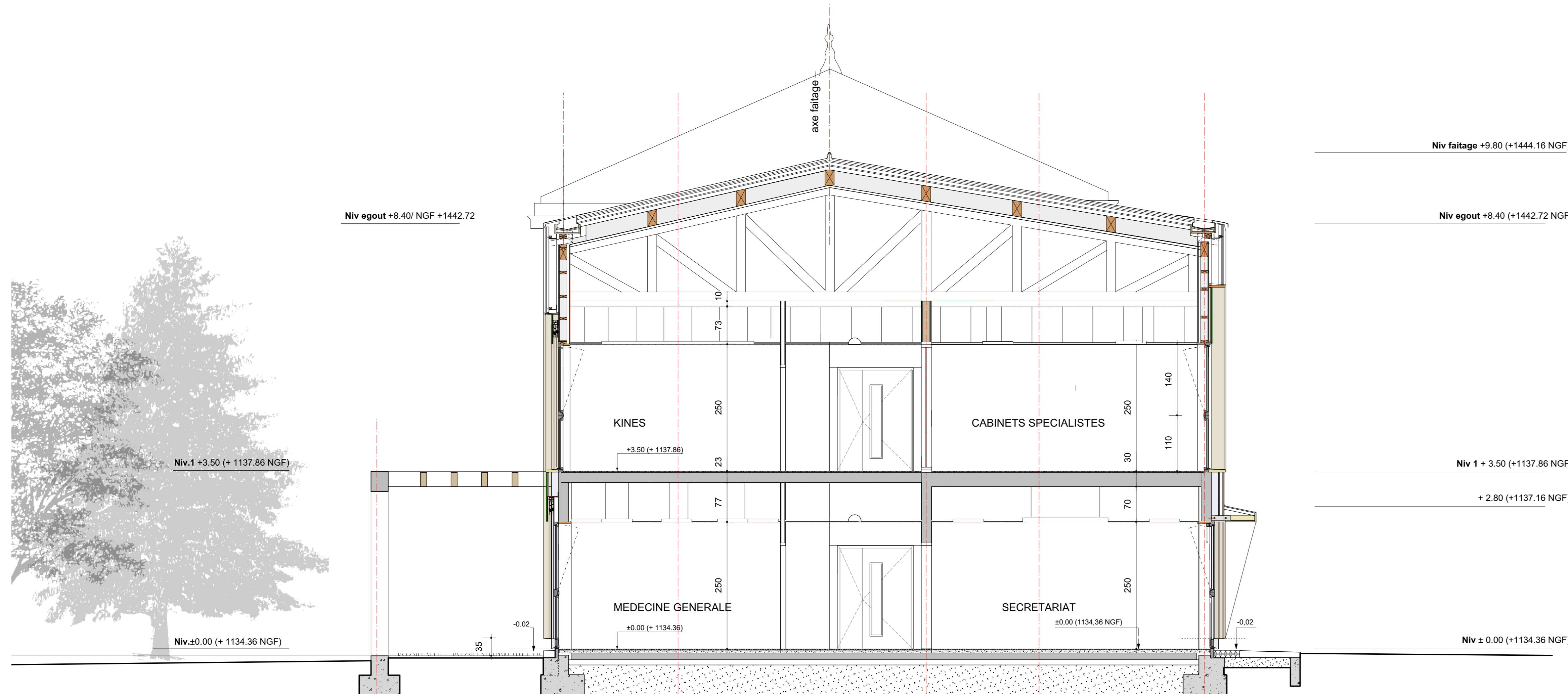
COUPE TRANSVERSALE SUR CABINET DENTISTE
