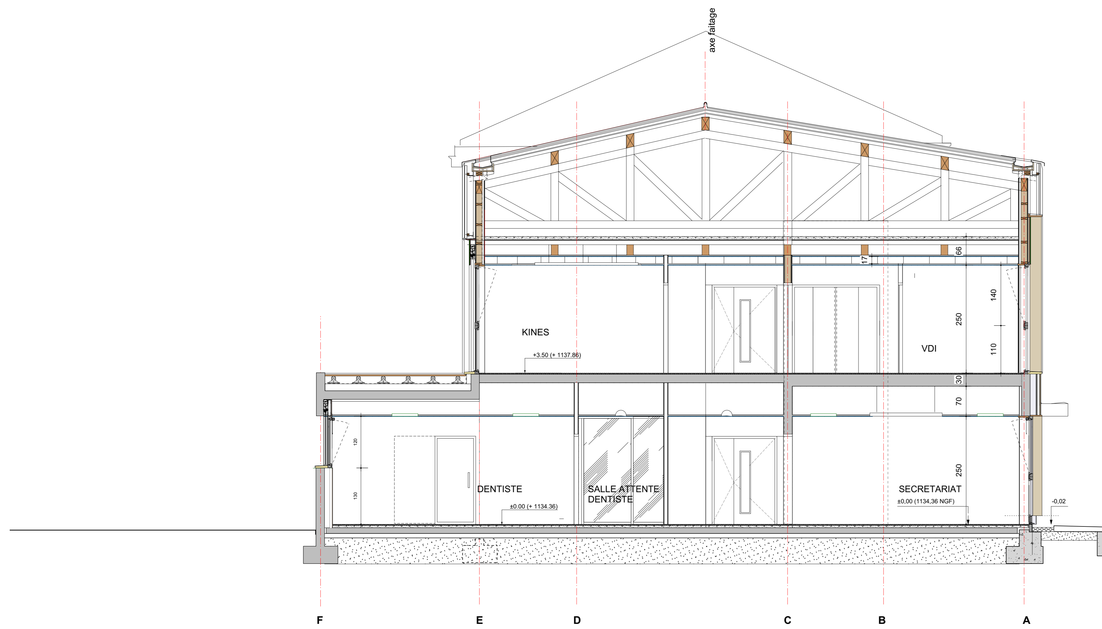
COUPE TRANSVERSALE SUR CABINET DENTISTE
