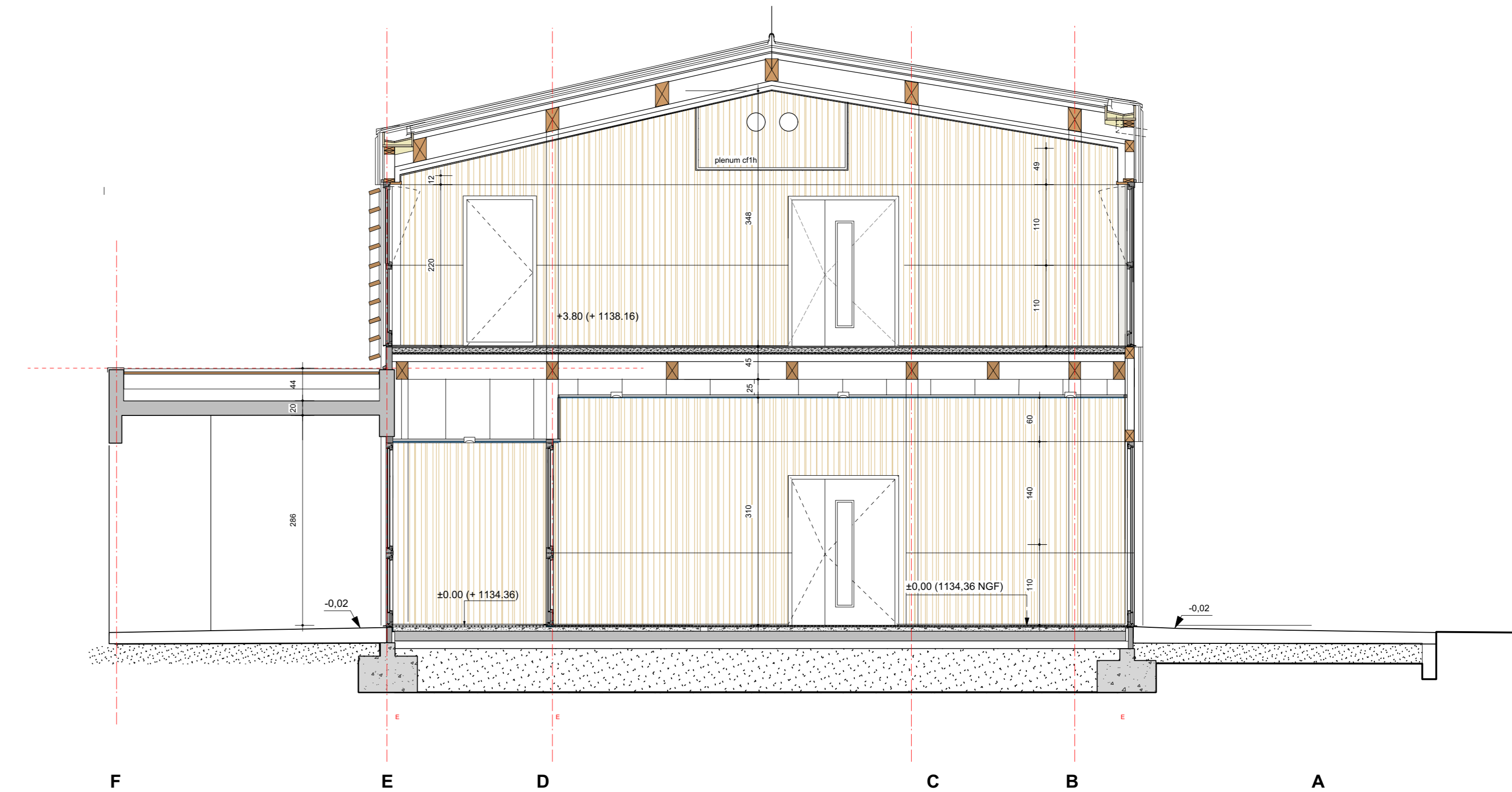
COUPE SUR ENTREE
