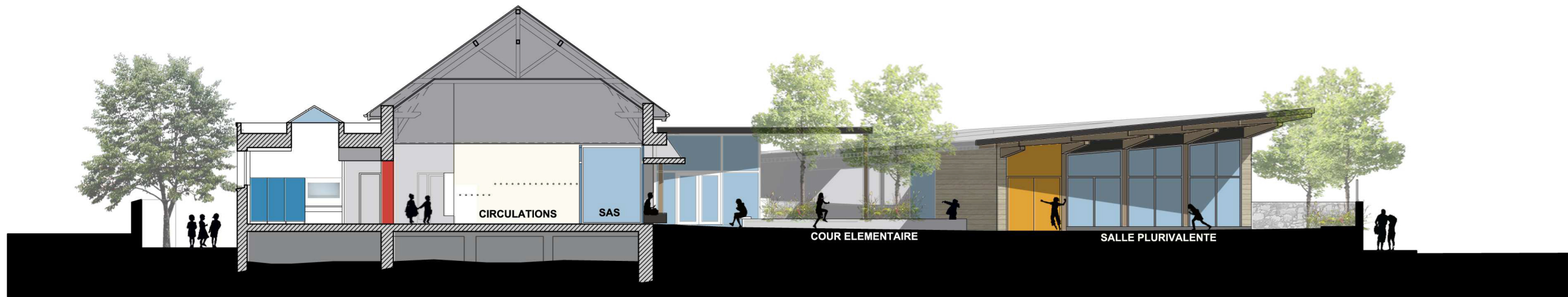
COUPE AA - SUR COUR ELEMENTAIRE
