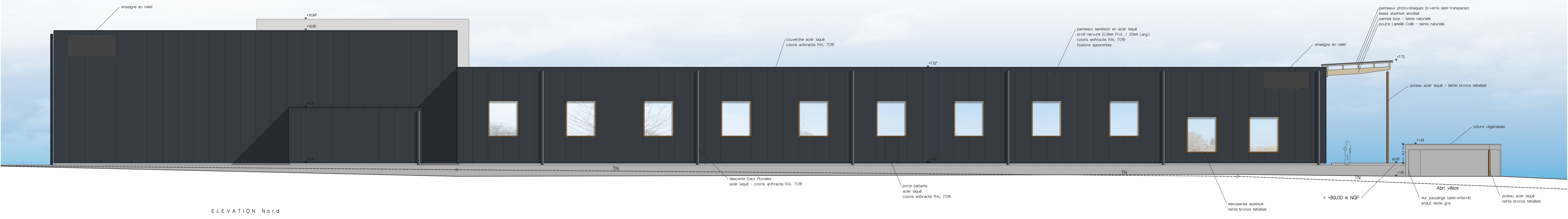
ELEVATION Nord
