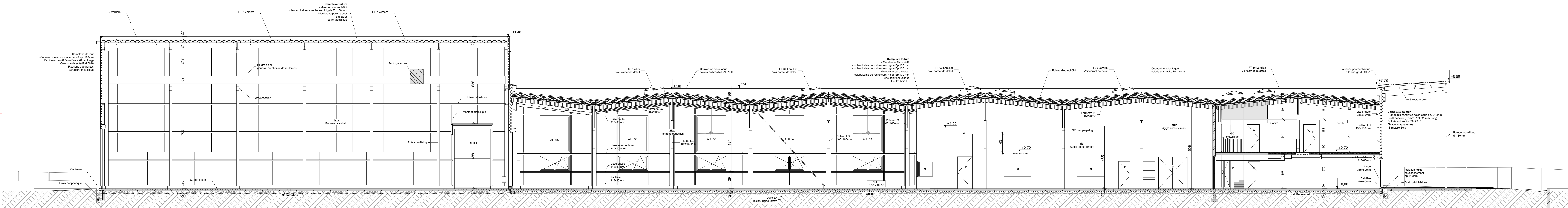
Coupe B-B'
