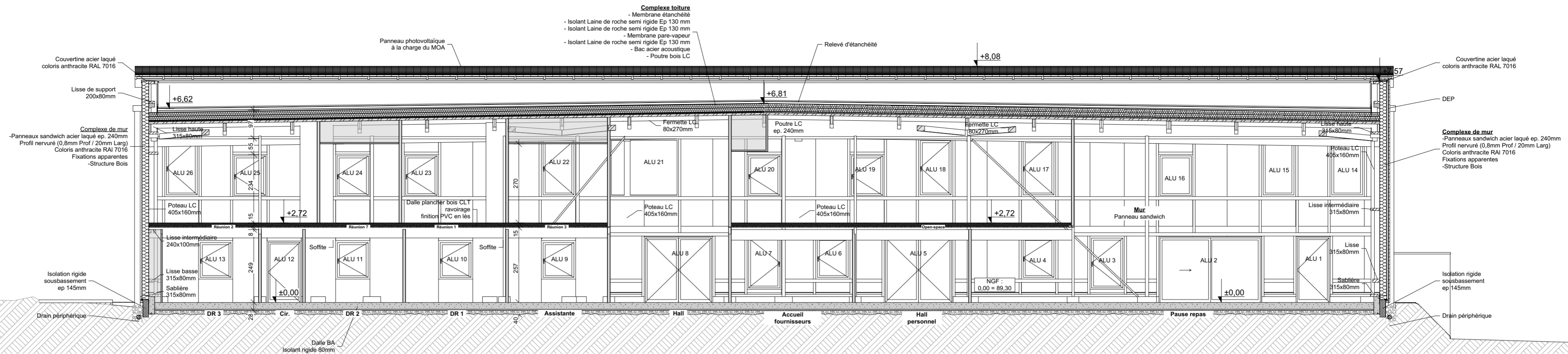
Coupe 1-1'
