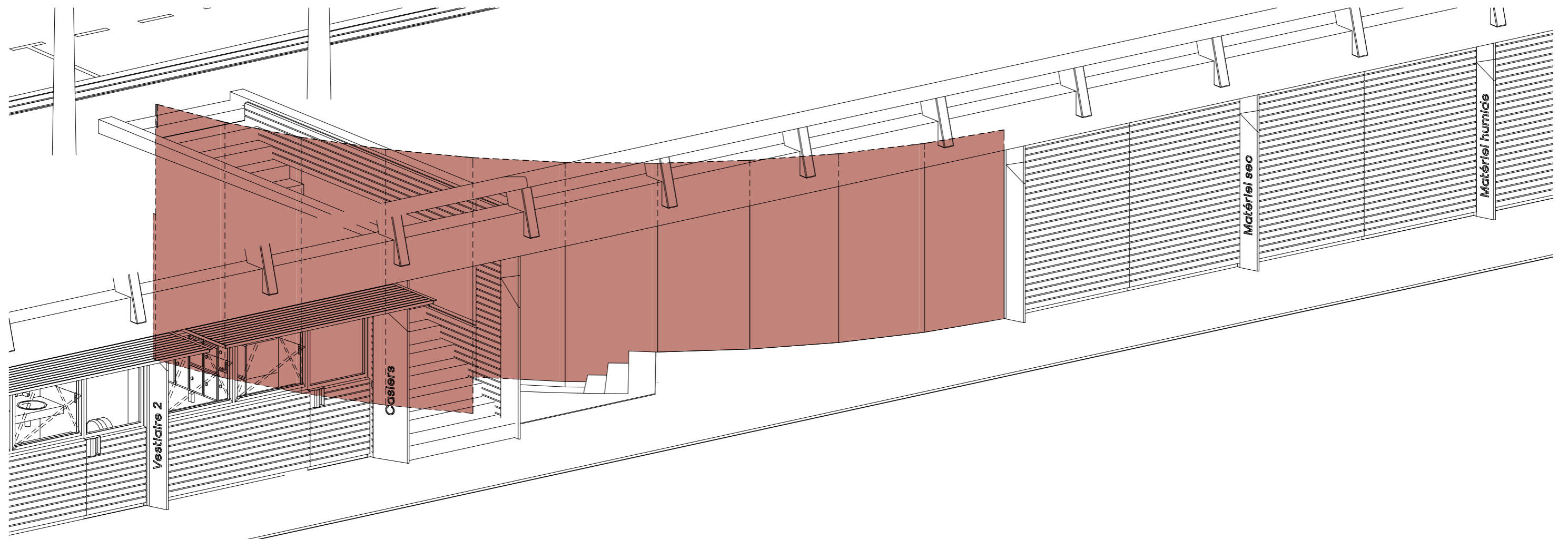
Base nautique de Golfe Juan - Détail mur en acier Cor-Ten 1:50
