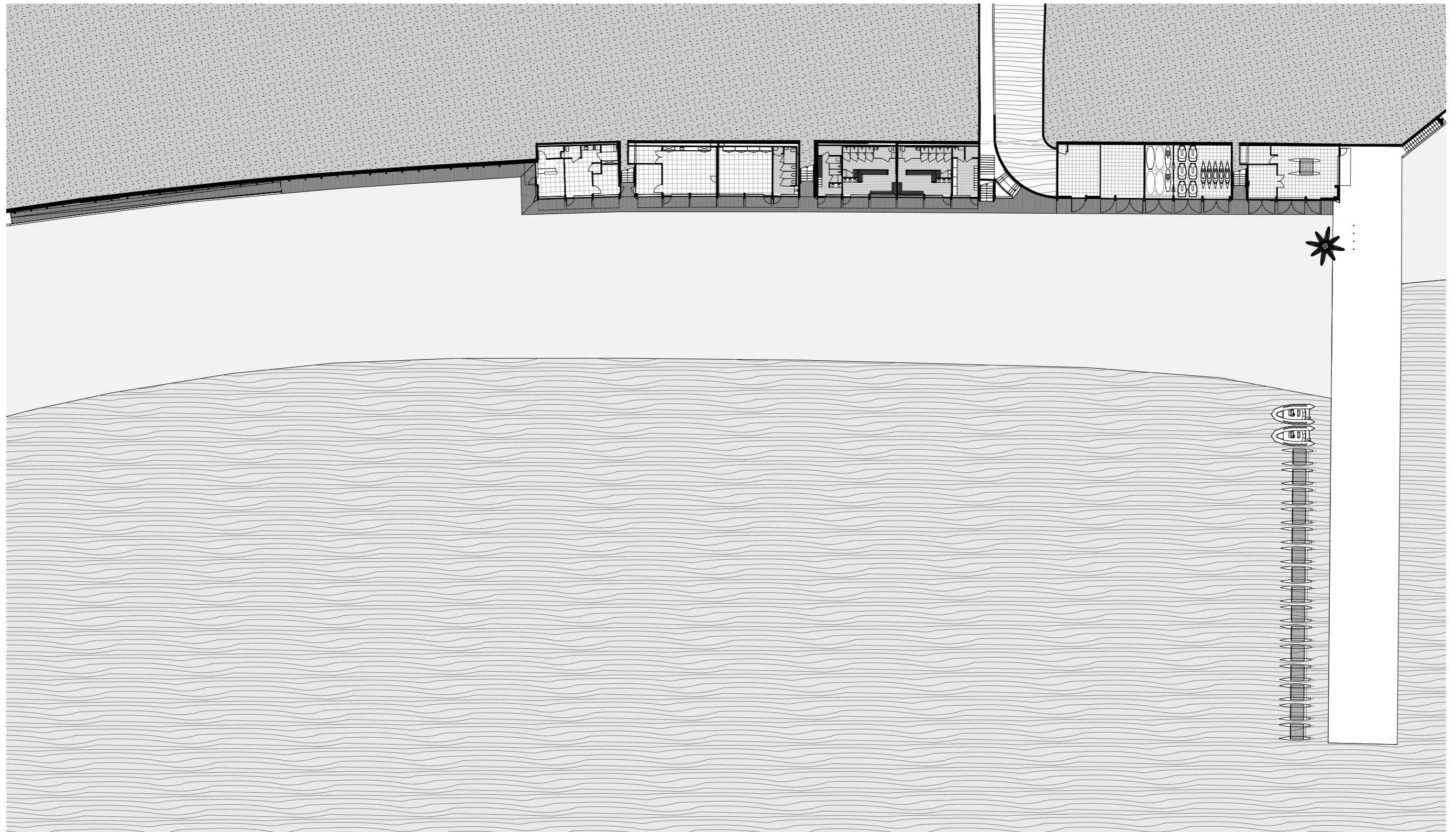
Base nautique de Golfe Juan - Plan 1:500
