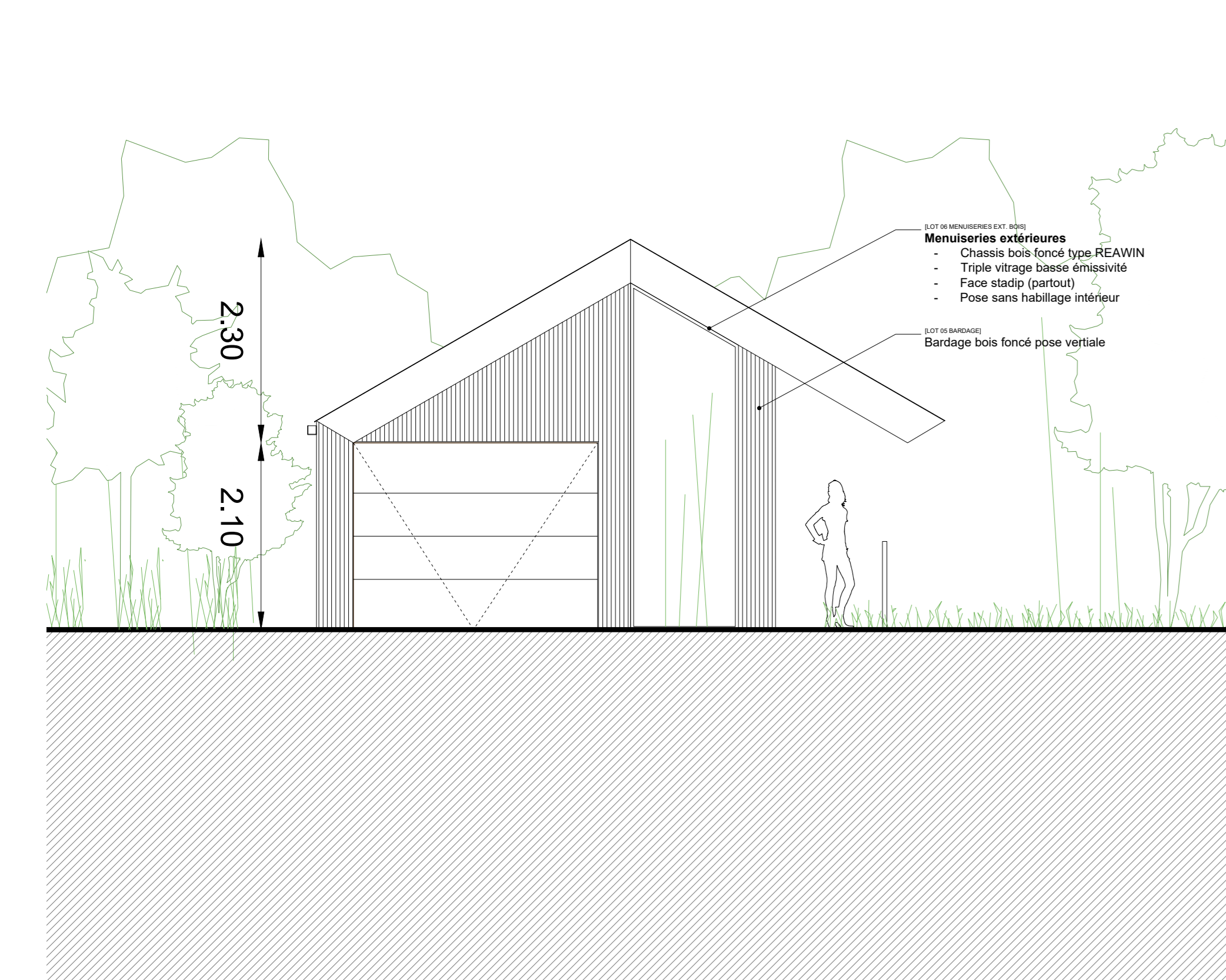
FAÇADE NORD
