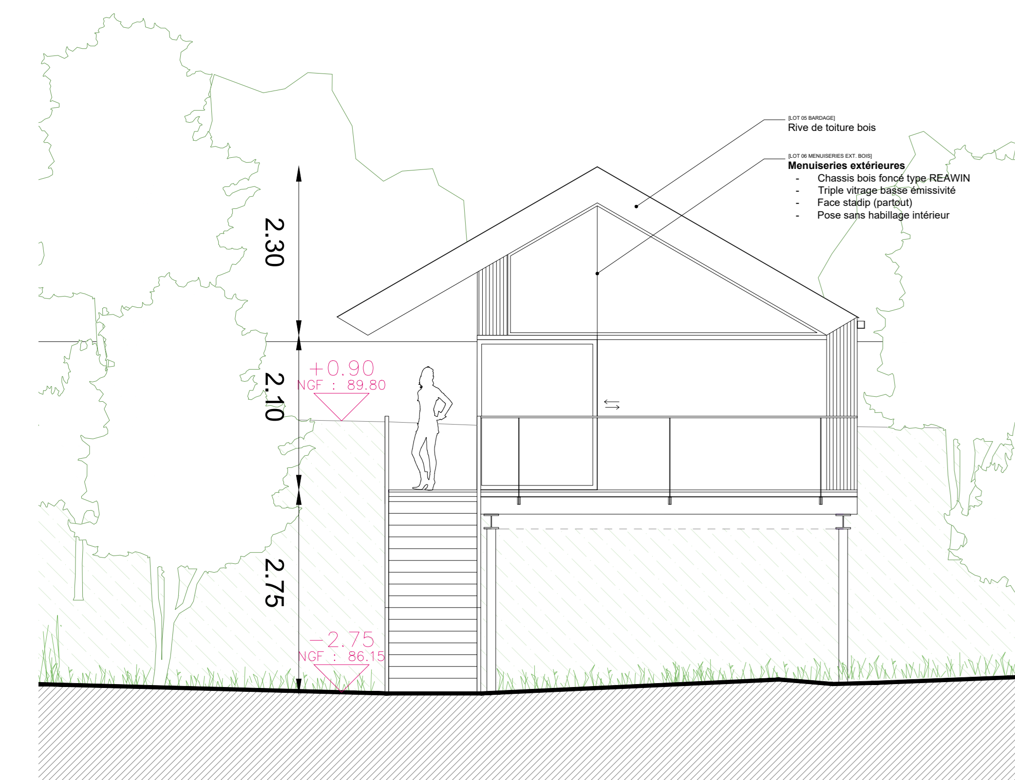
FAÇADE SUD
