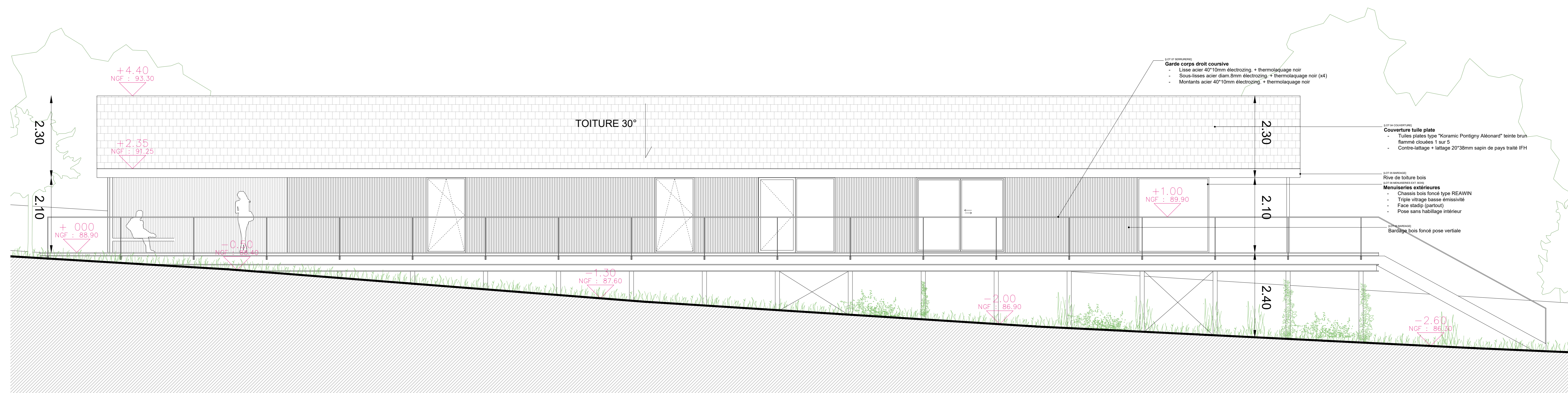
FAÇADE OUEST
