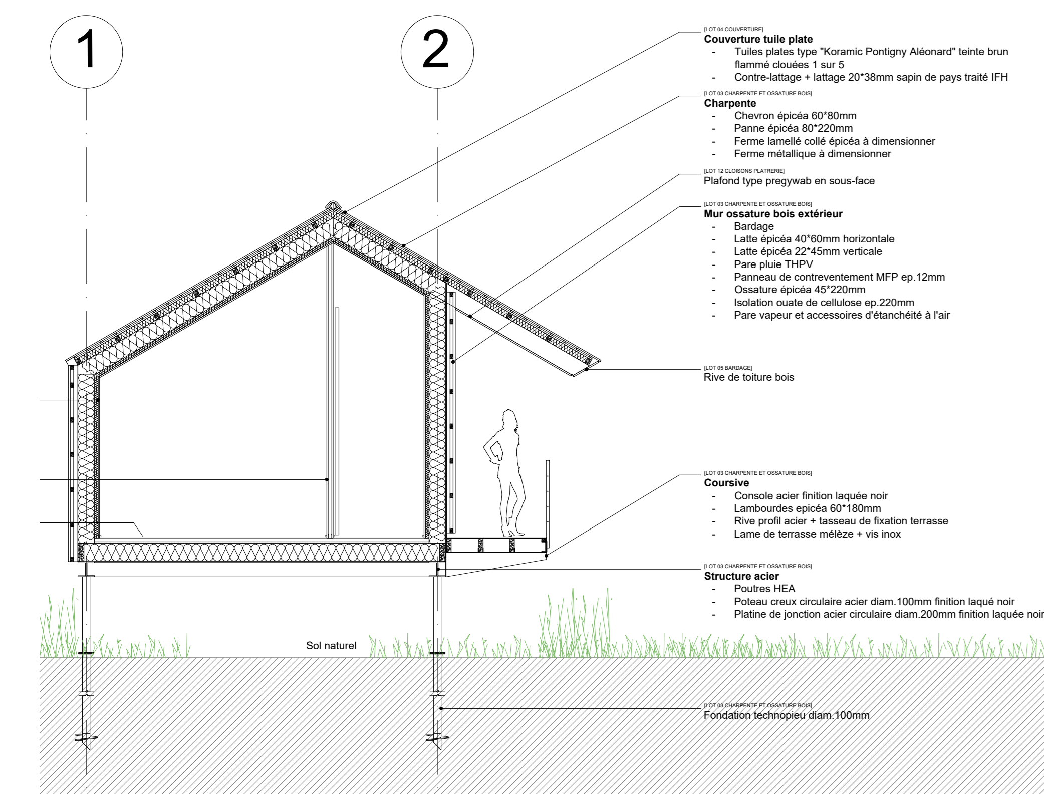
COUPE TRANSVERSALE
