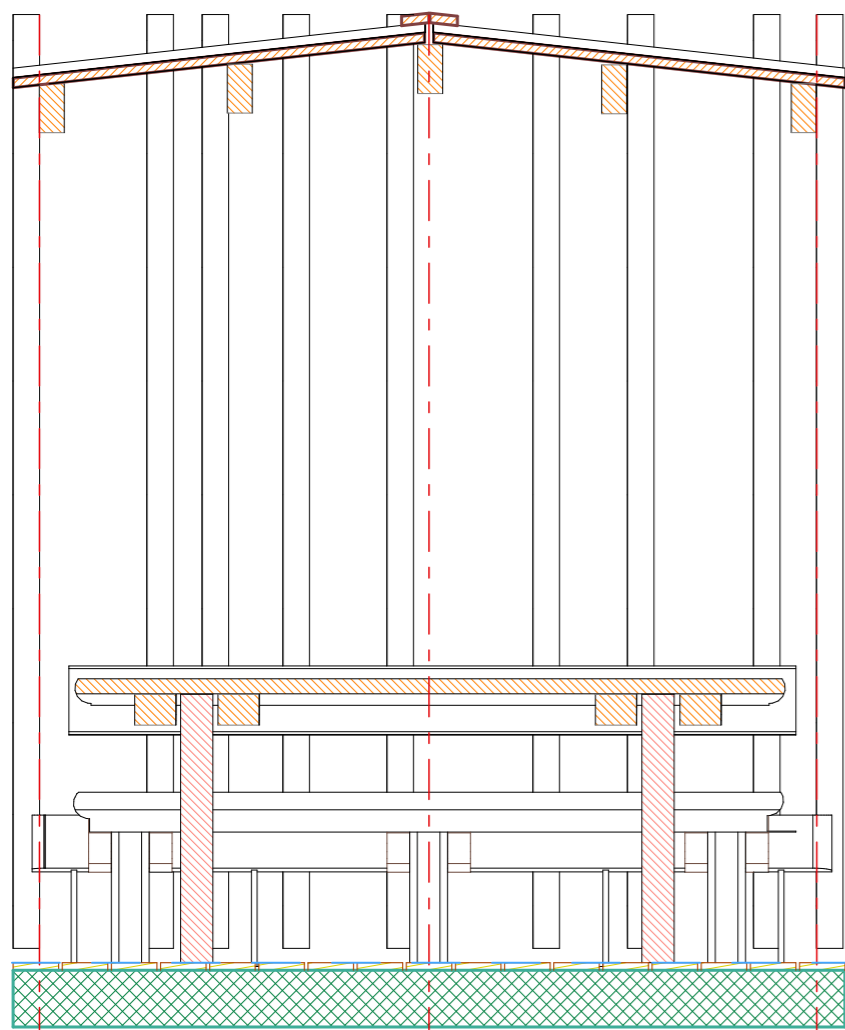
Coupe Longitudinale de principe
