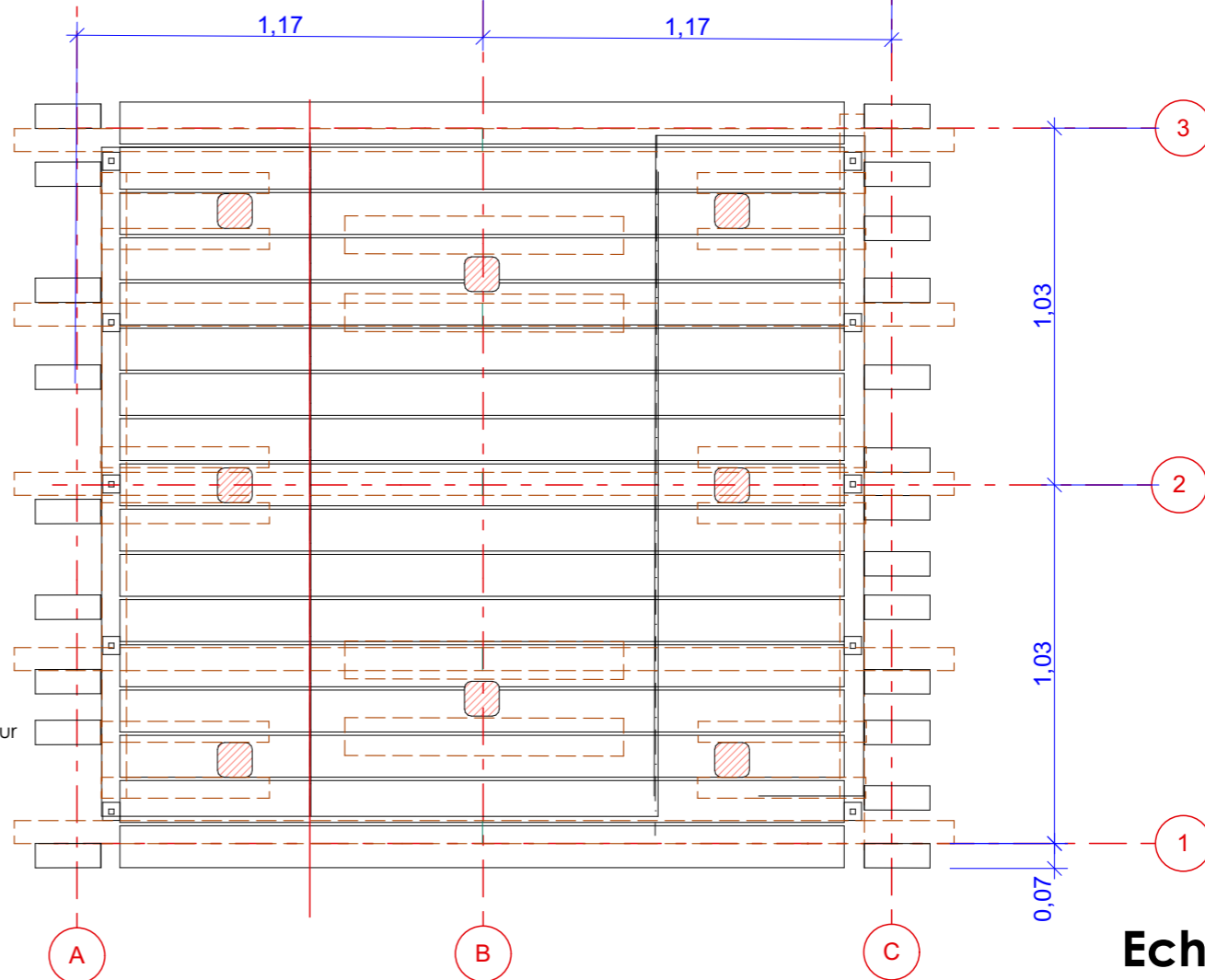
Coupe Transversale de principe
