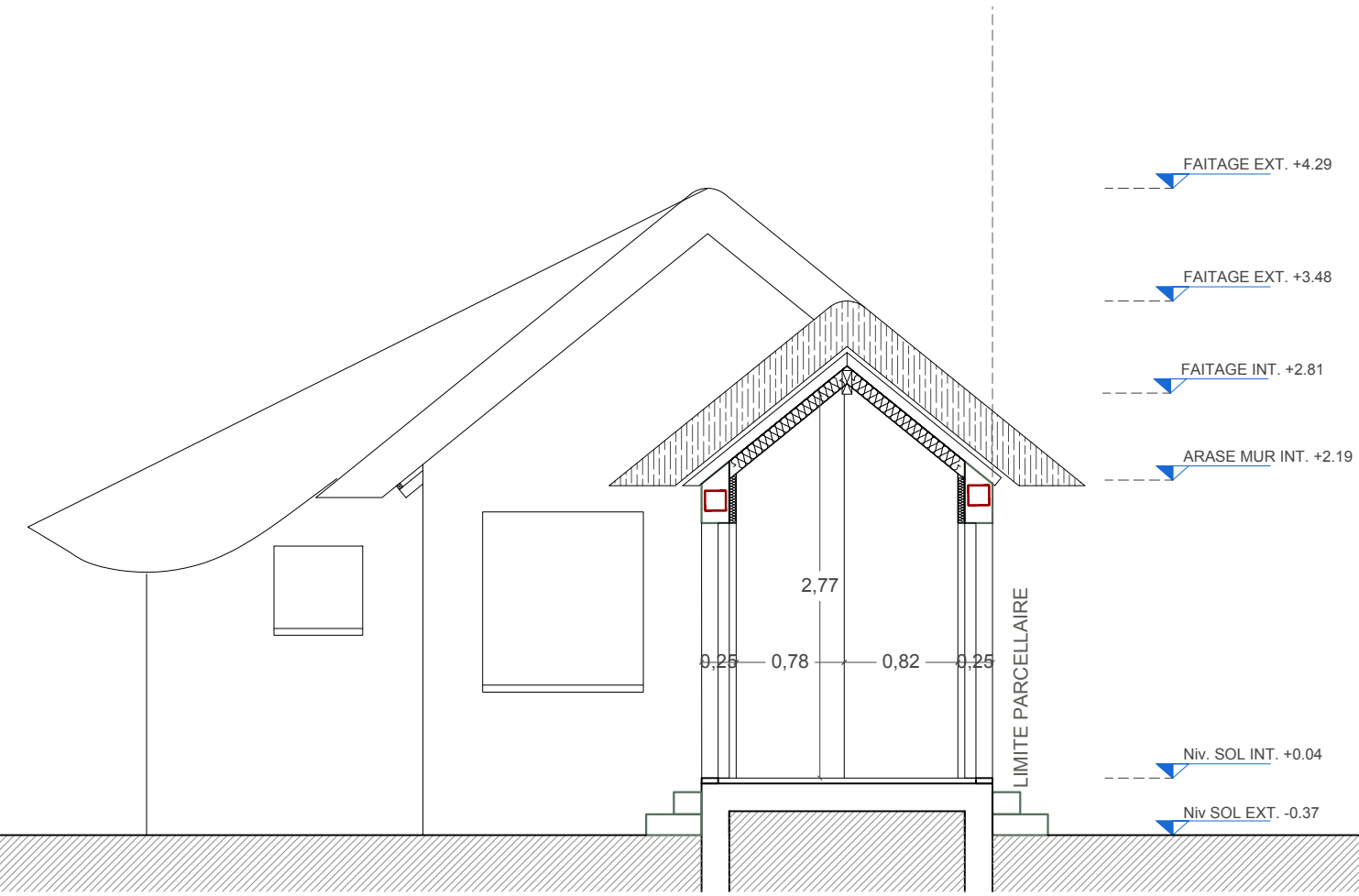
COUPE AA
