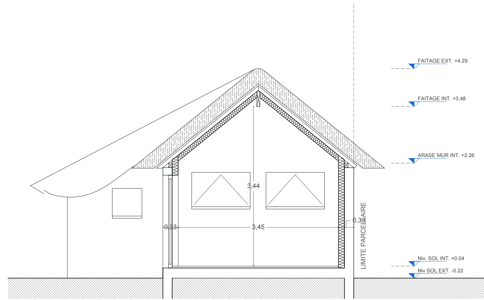
COUPE BB
