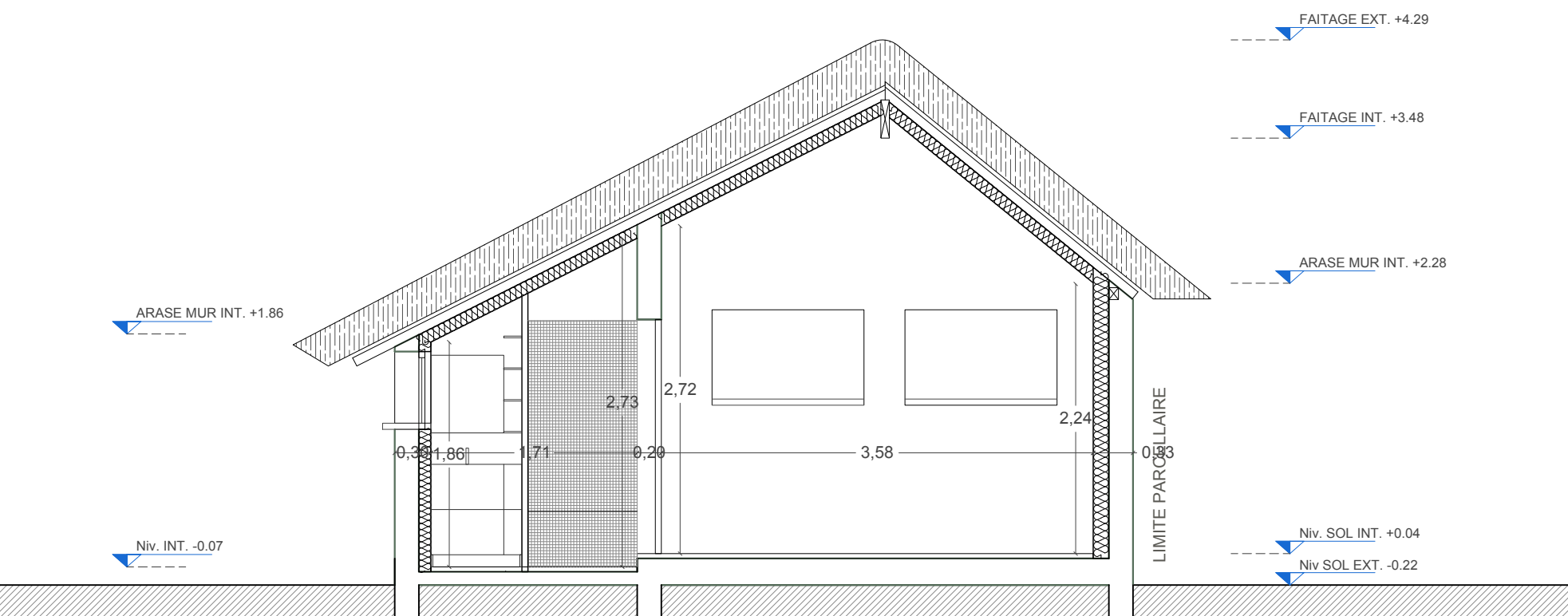
COUPE CC
