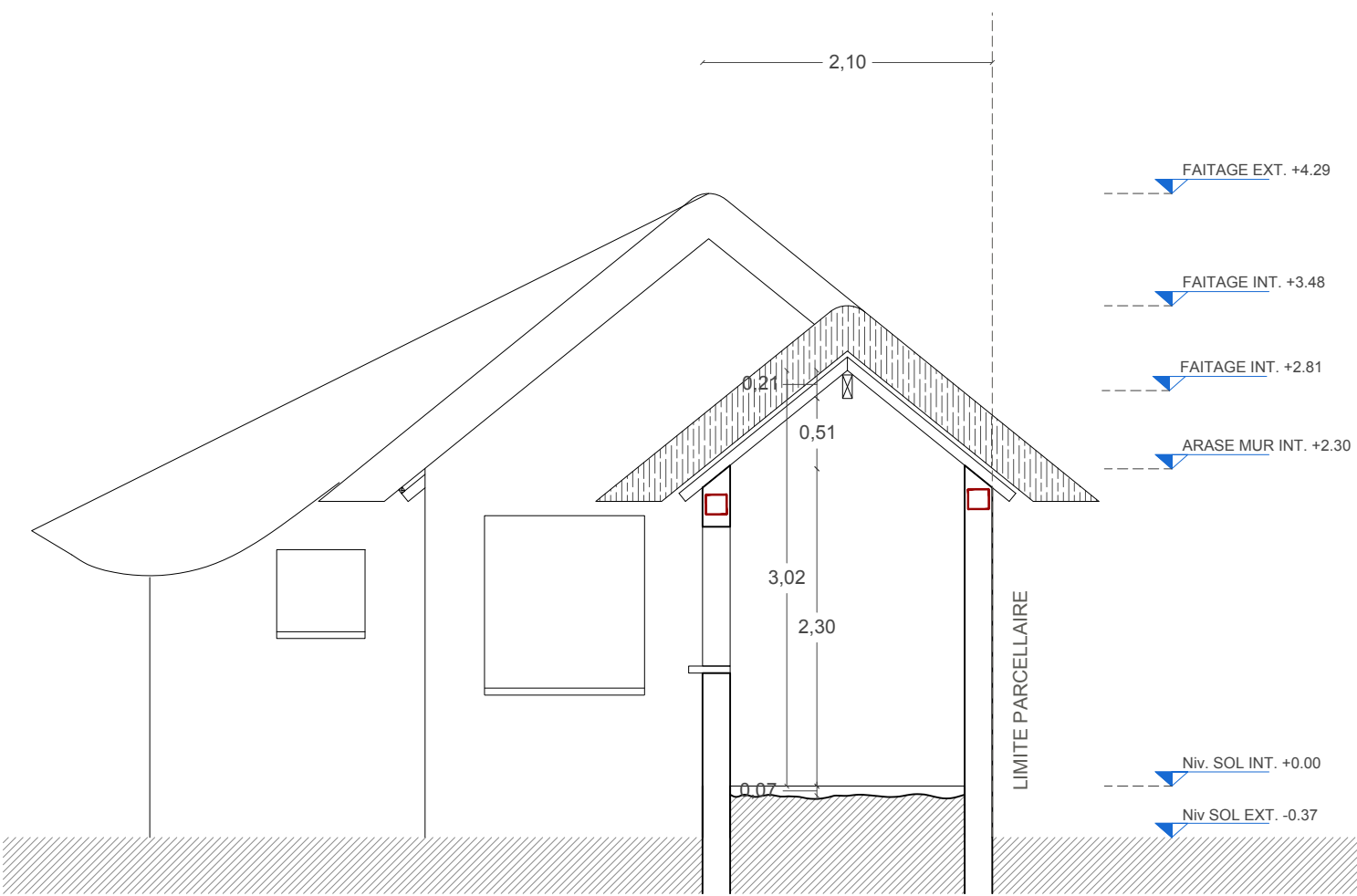
COUPE AA
