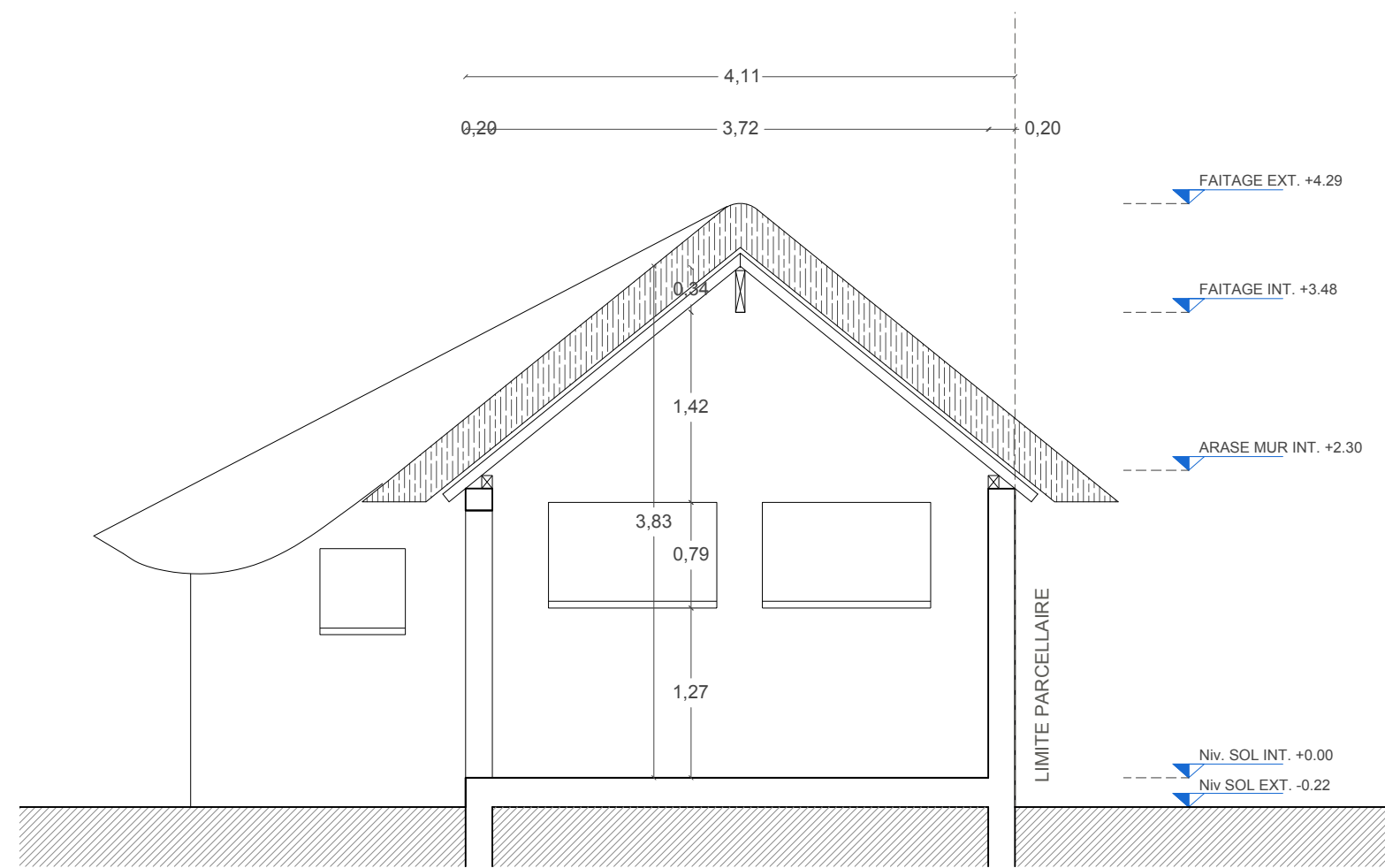
COUPE BB
