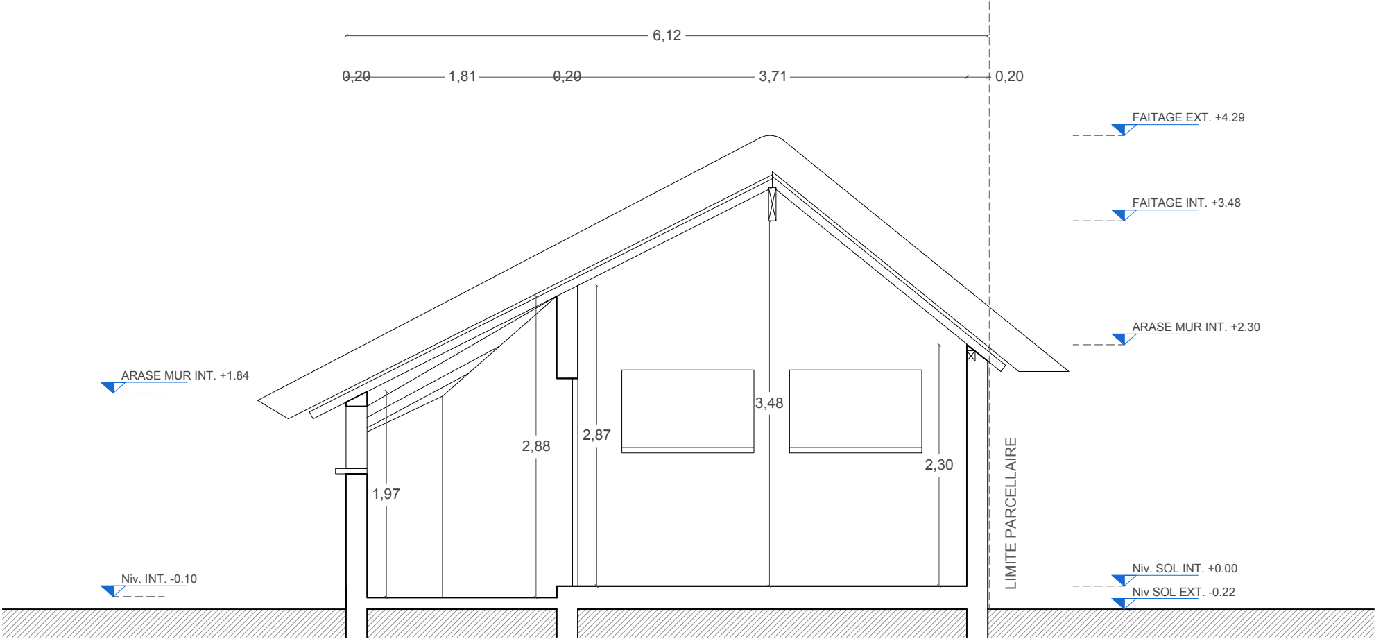
COUPE CC
