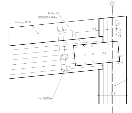
Détail A7: Assemblage Poteau/Arbalétrier courant
