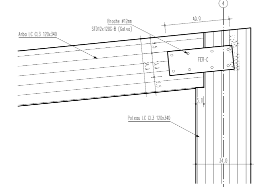
Détail A6: Assemblage Poteau/Arbalétrier en pignon
