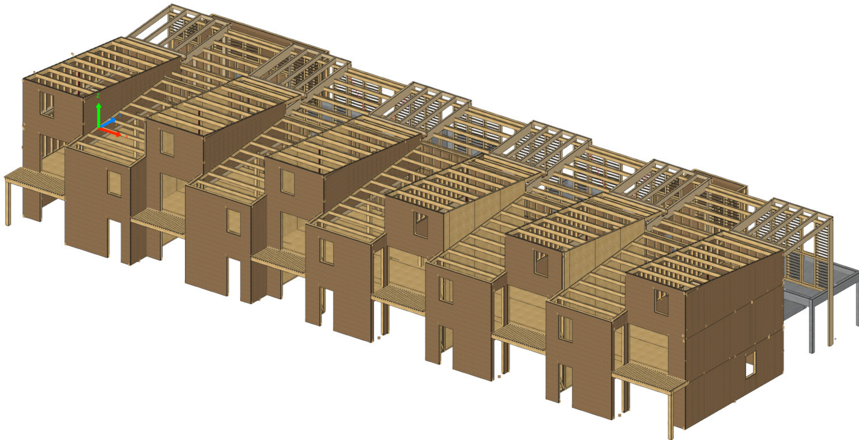
AXONOMETRIE SUD (vue des logements et balcons)
