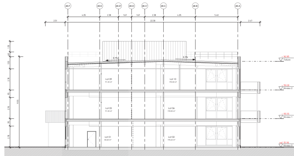
2 Coupe BB Ech : 1 : 100
