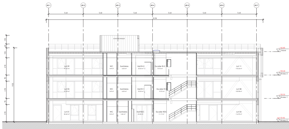
3 Coupe CC Ech : 1 : 100
