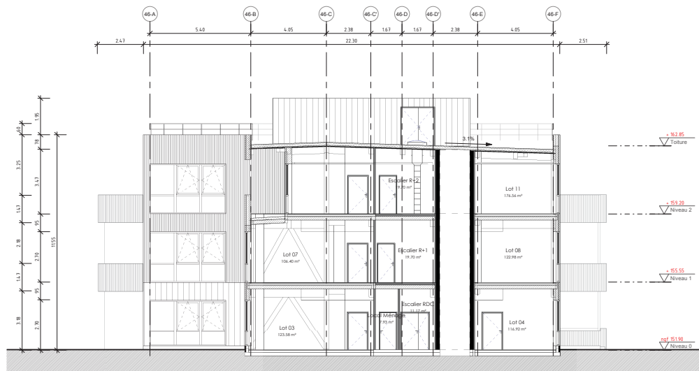
1 Coupe AA Ech : 1 : 100
