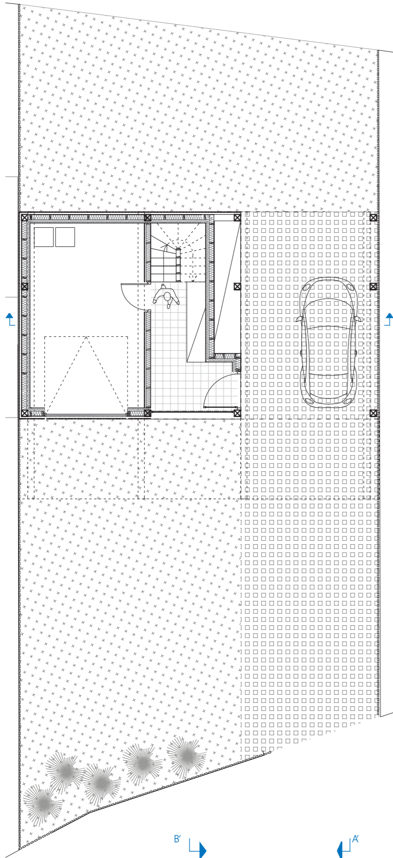
PLAN RDC.
