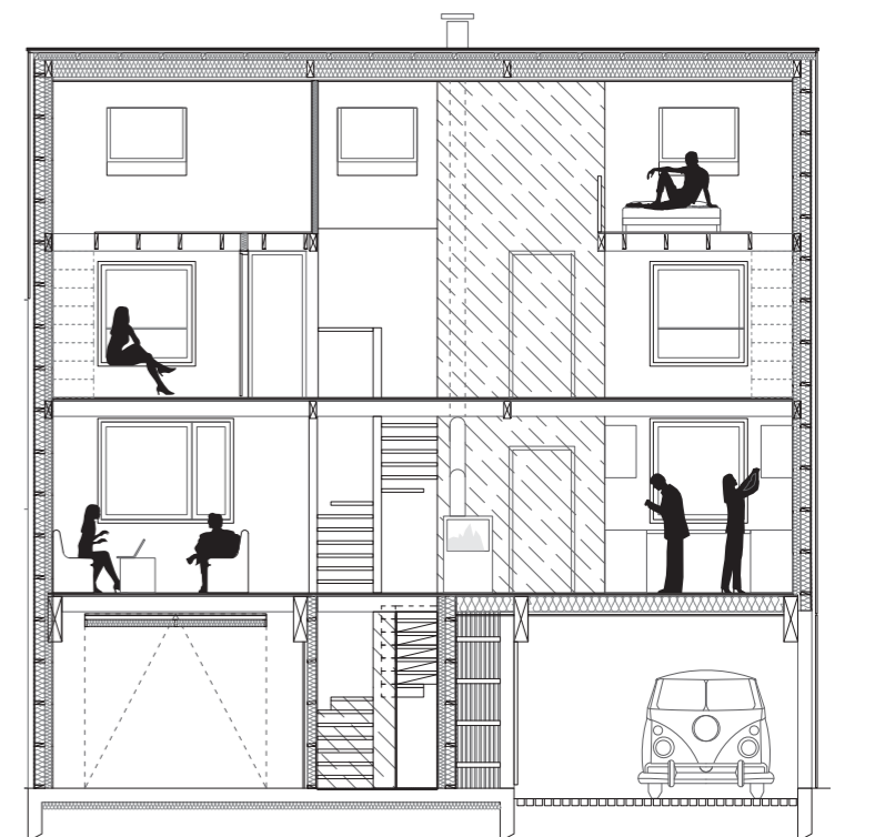
COUPE LONGITUDINALE
