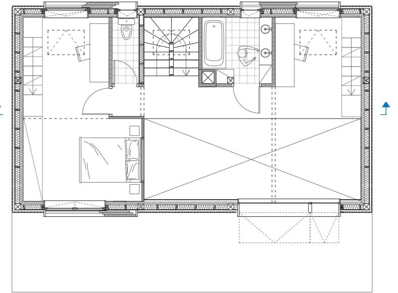
PLAN R+2
