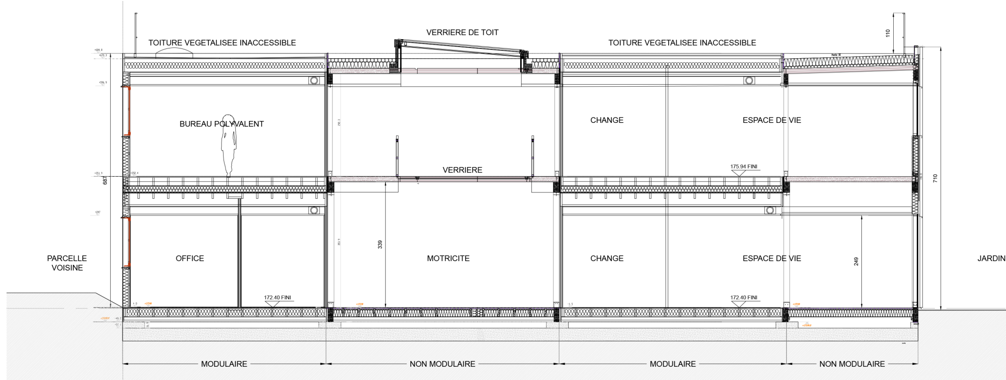
COUPE TRANSVERSALE AA ECH 1/100
