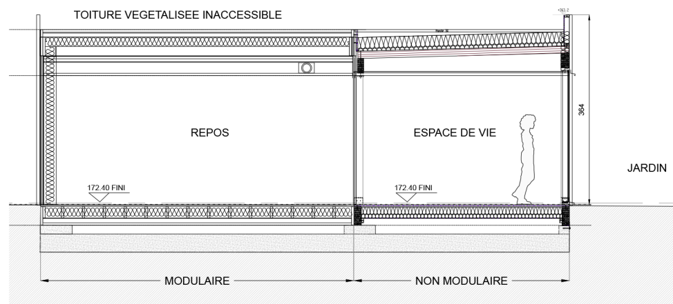
COUPE TRANSVERSALE BB ECH 1/100
