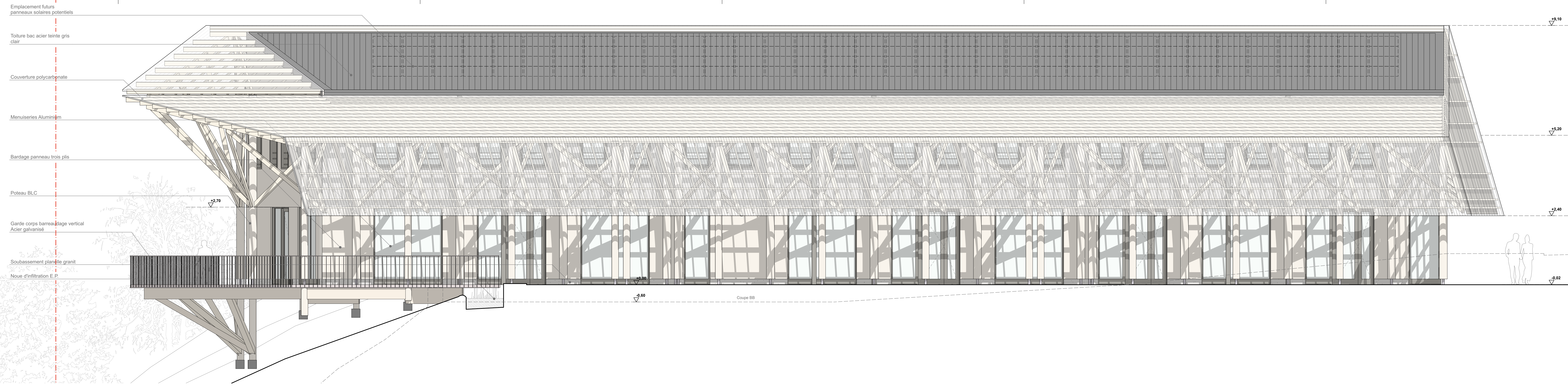
Façade Sud Halle
