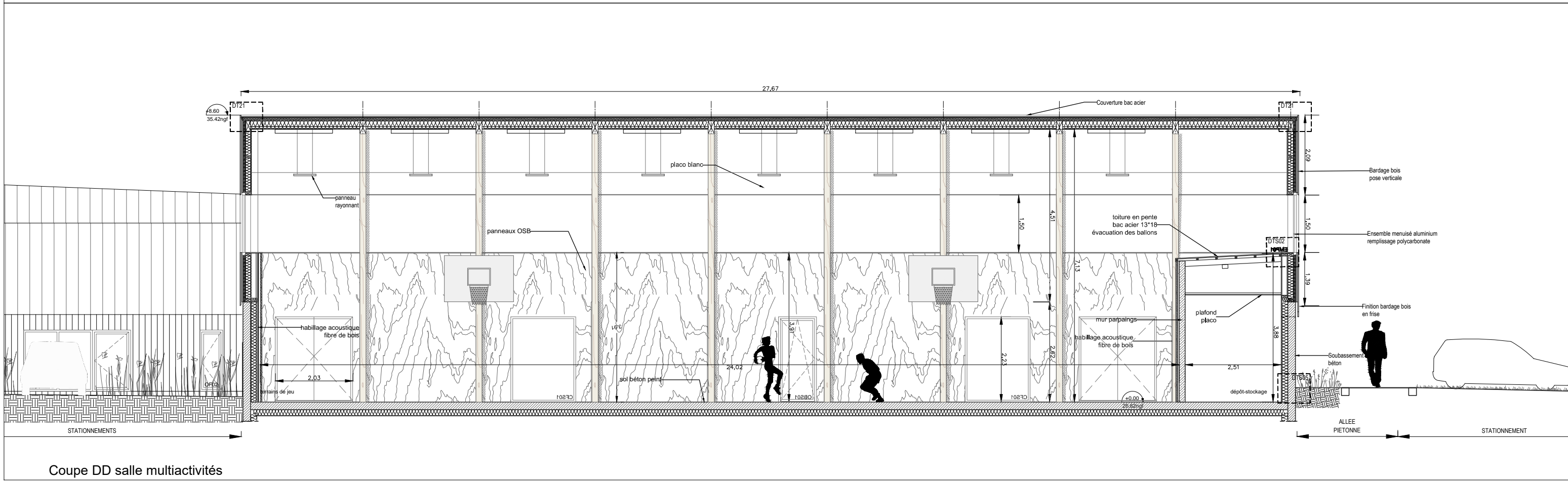
Coupe AA salle multiactivités
