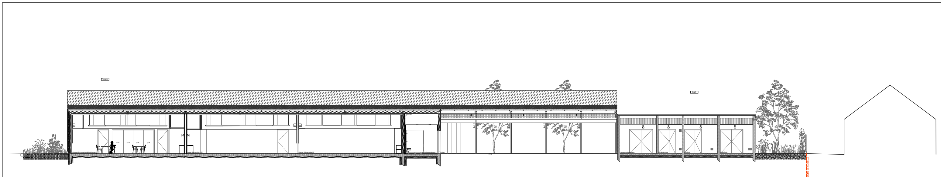
Coupe EE école
