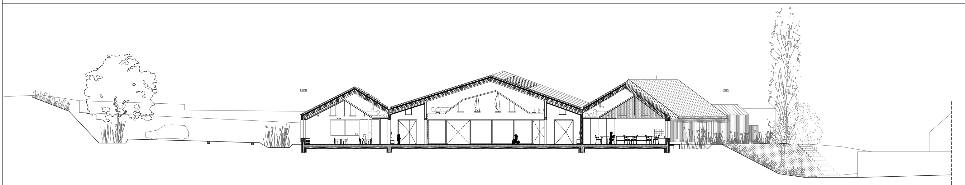
Coupe BB école
