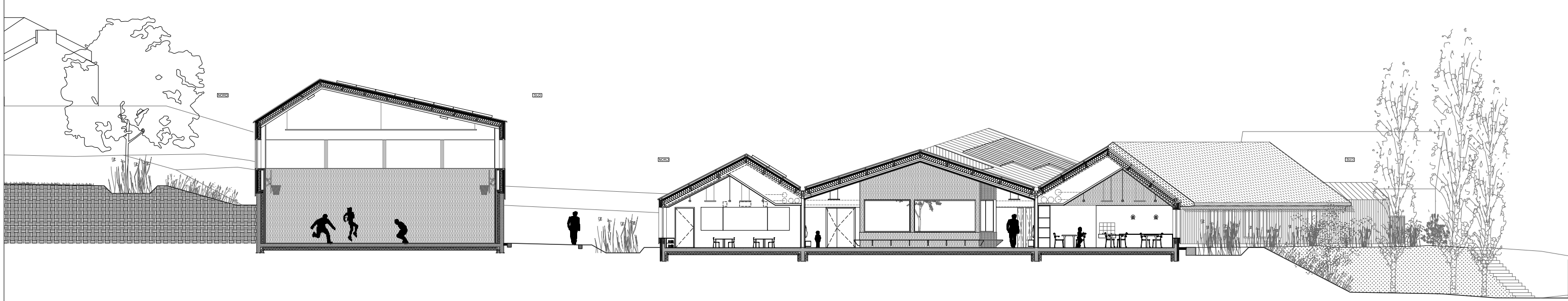
Coupe AA salle + école
