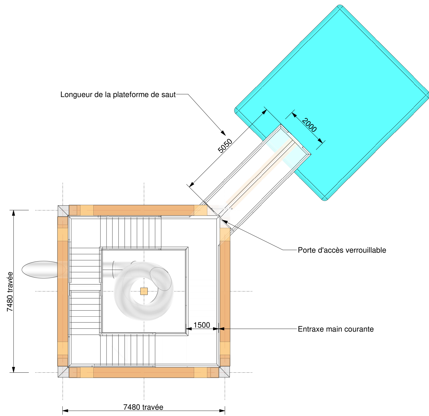
Vue en Plan au niveau de la plateforme de saut
