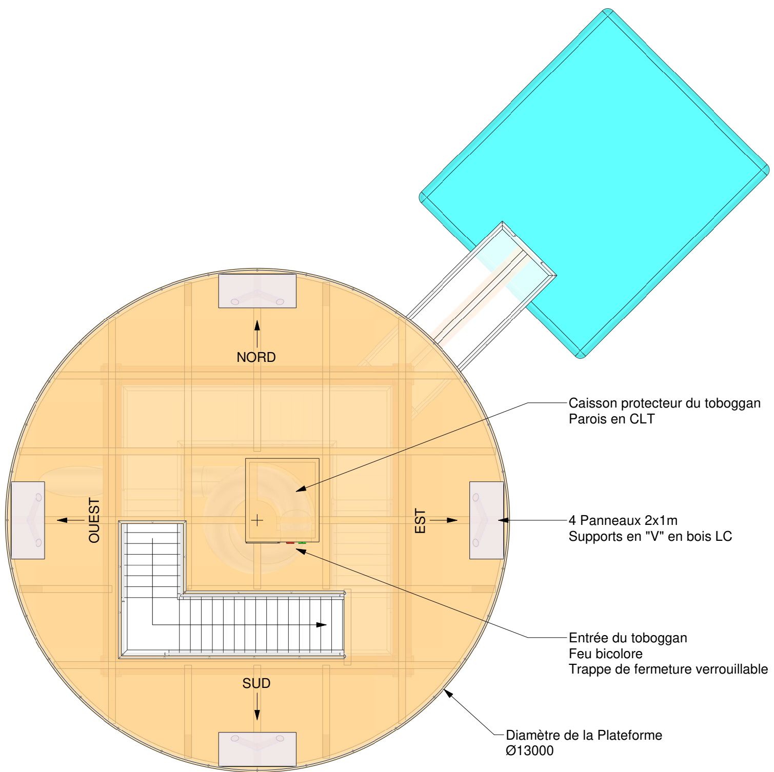
Vue en Plan au niveau de la plateforme sommitale
