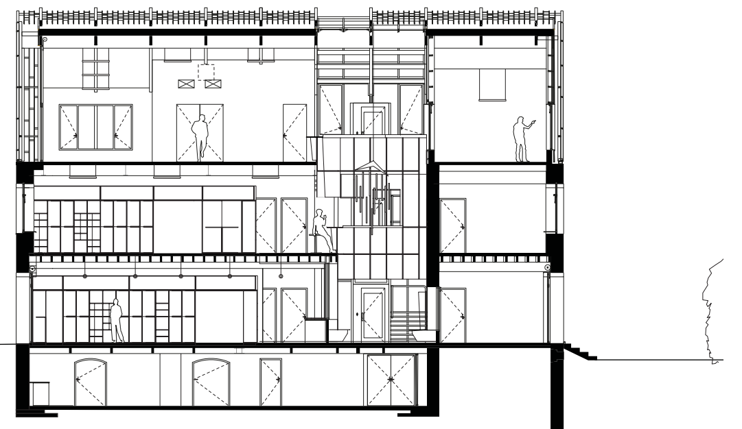
COUPE LONGITUDINALE
