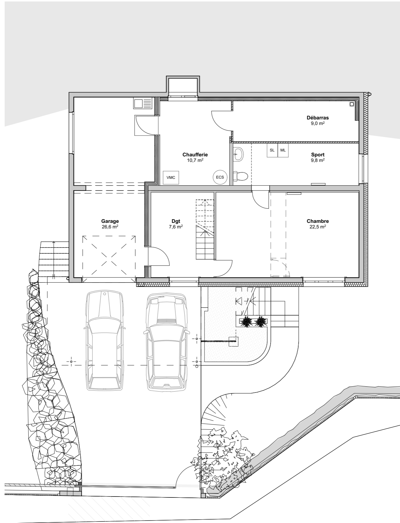
Plan du niveau bas
