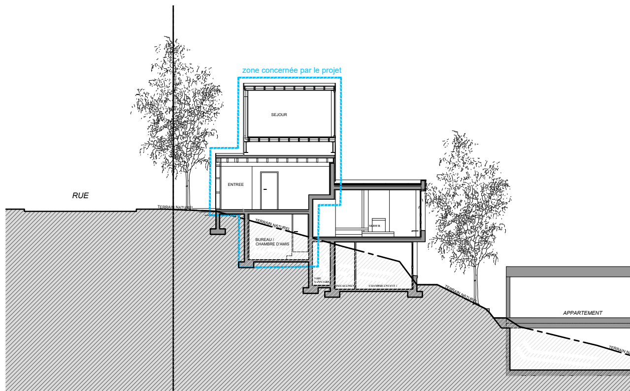
COUPE BB
