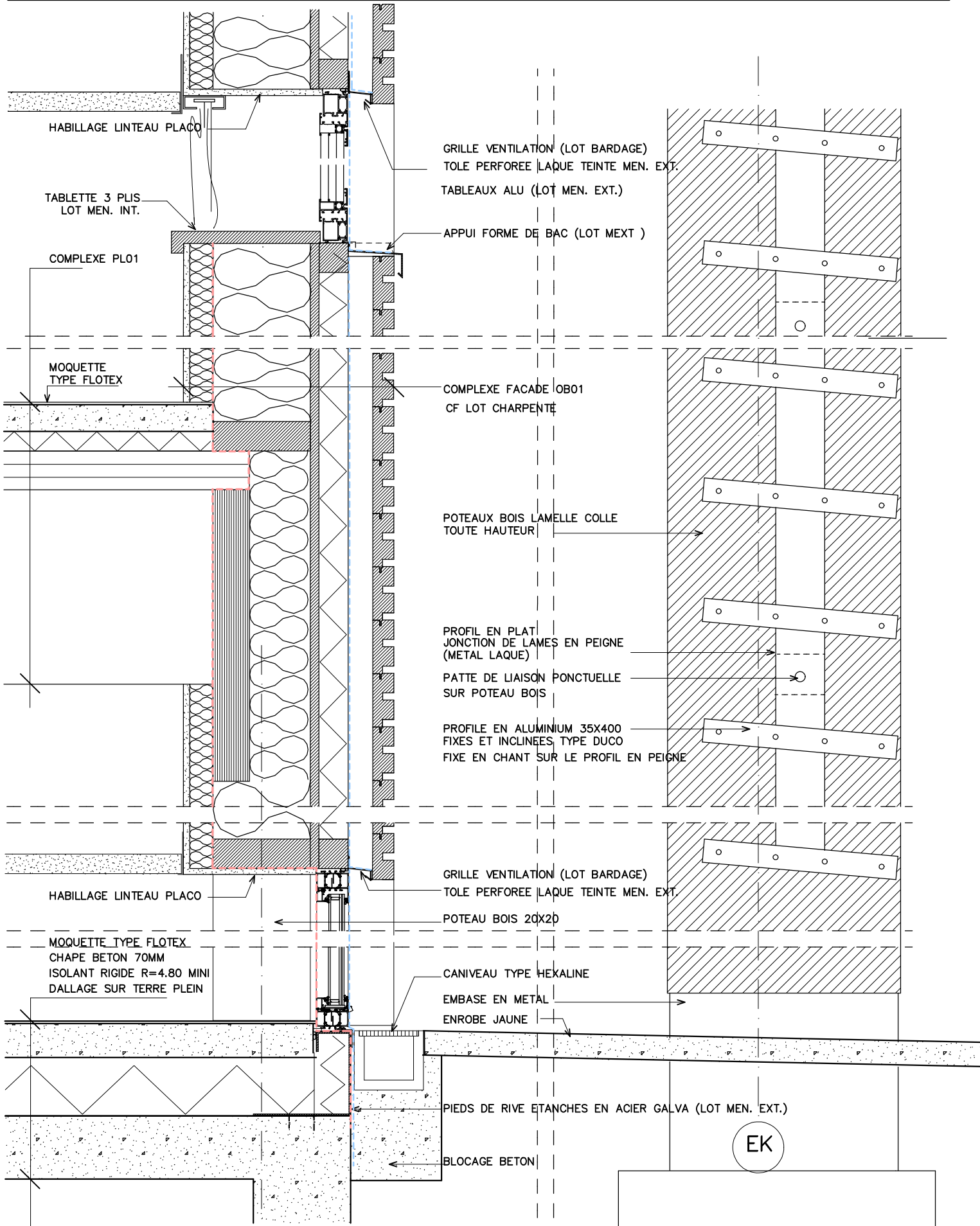
COUPE VERT. SUR CHASSIS FACADE SUD
