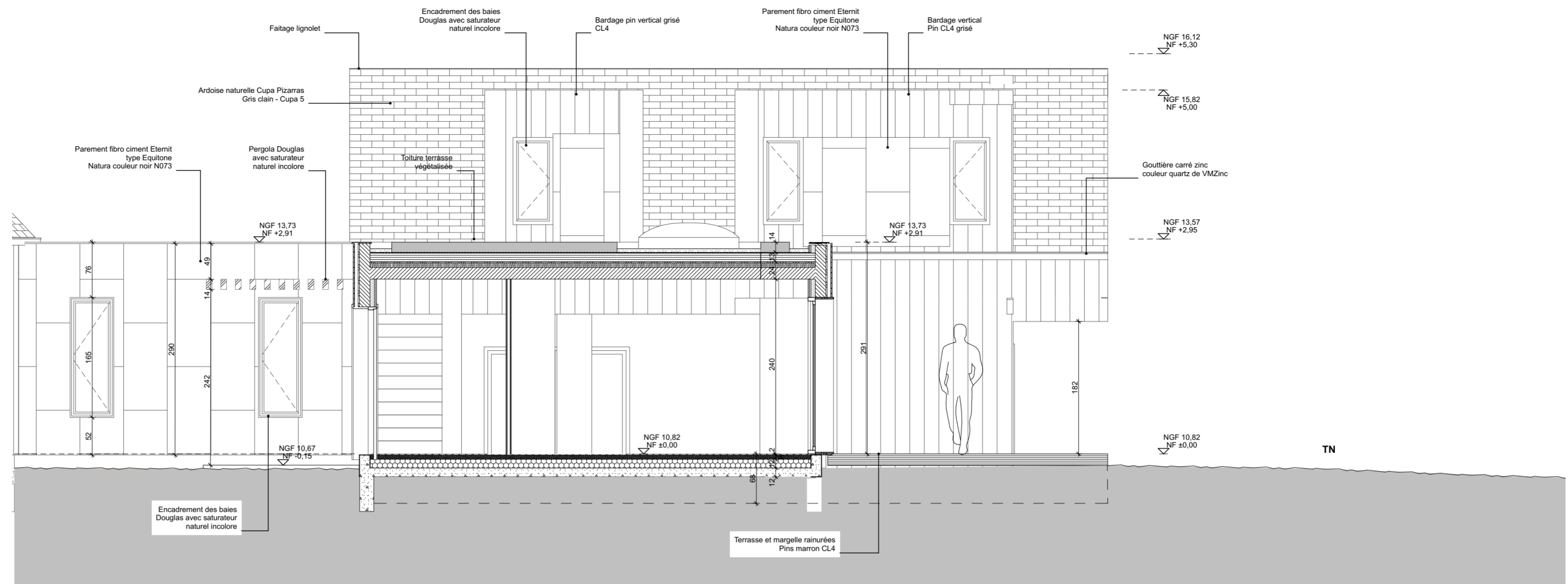
Coupe BB
