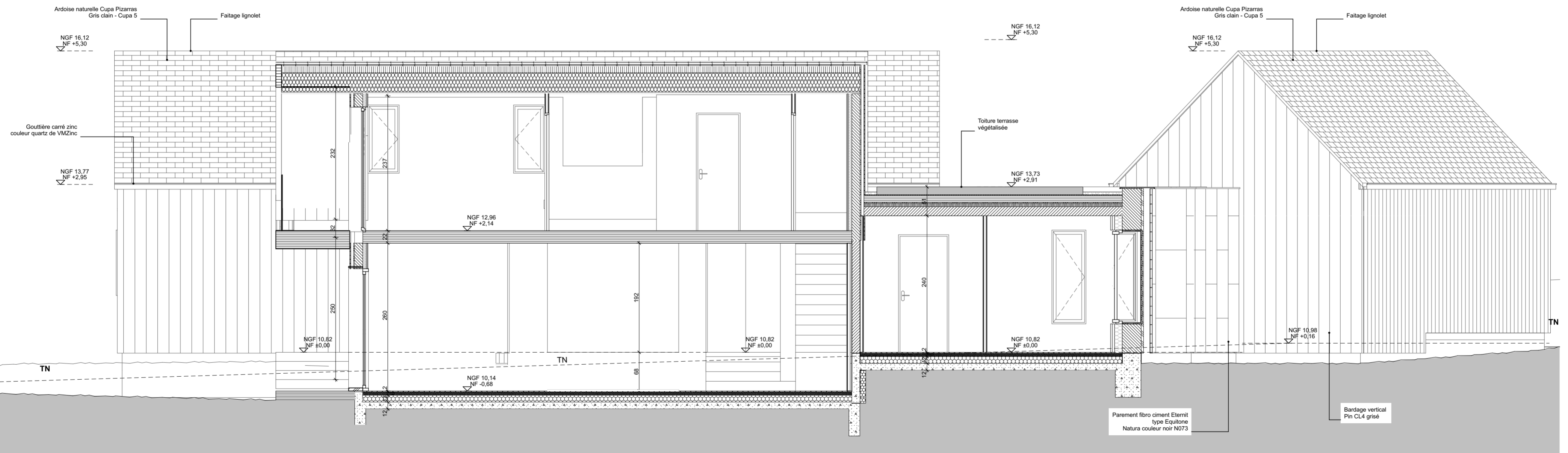
Coupe CC
