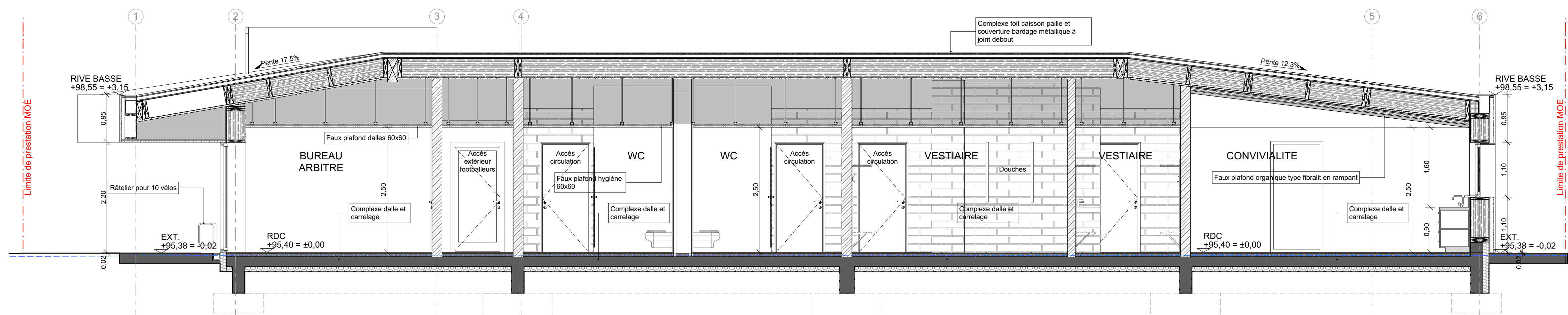
COUPE CC 1/50
