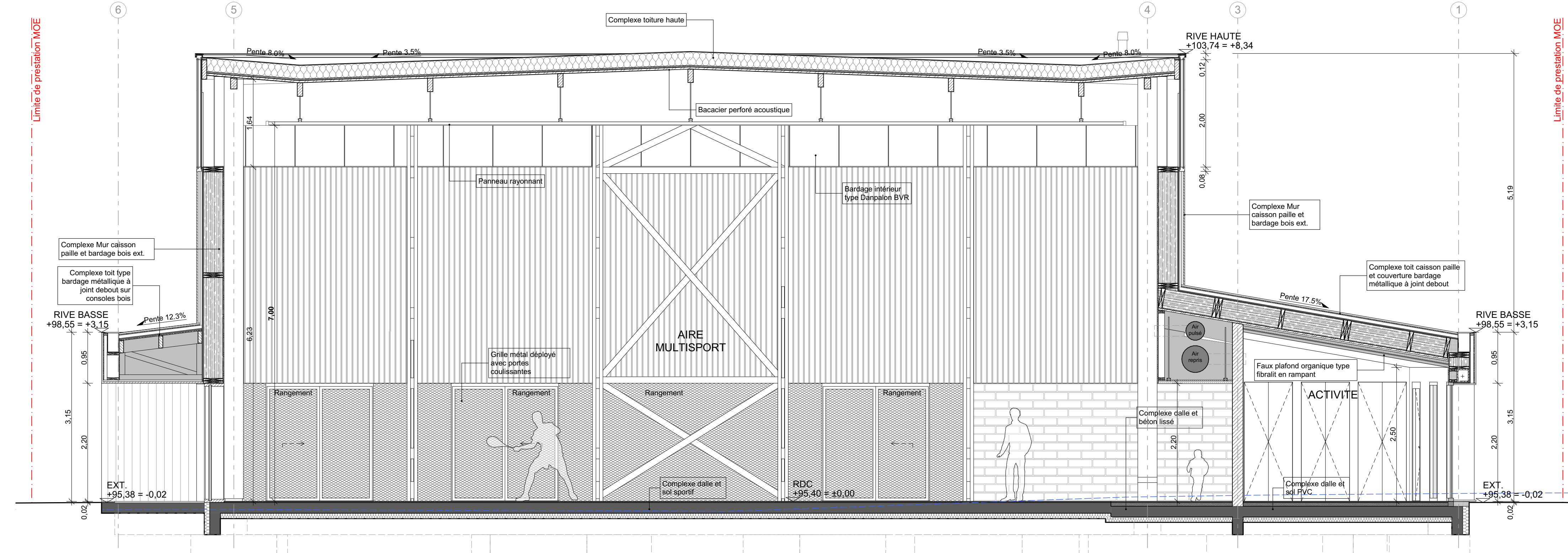
COUPE EE 1/50
