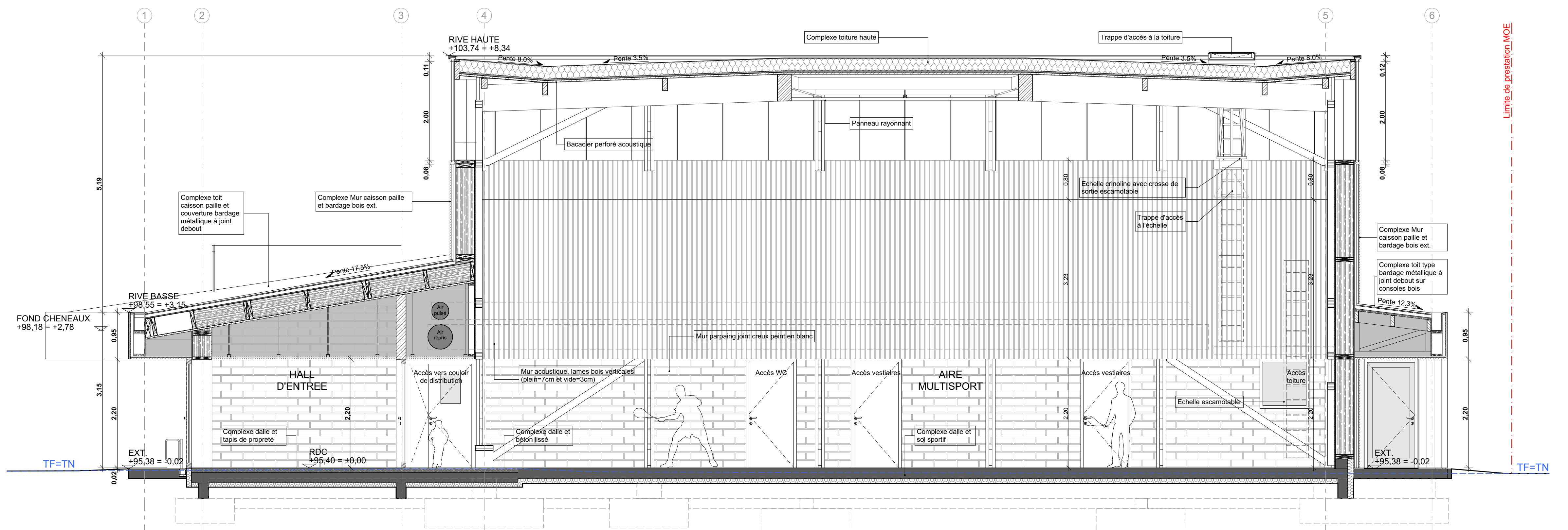
COUPE AA 1/50
