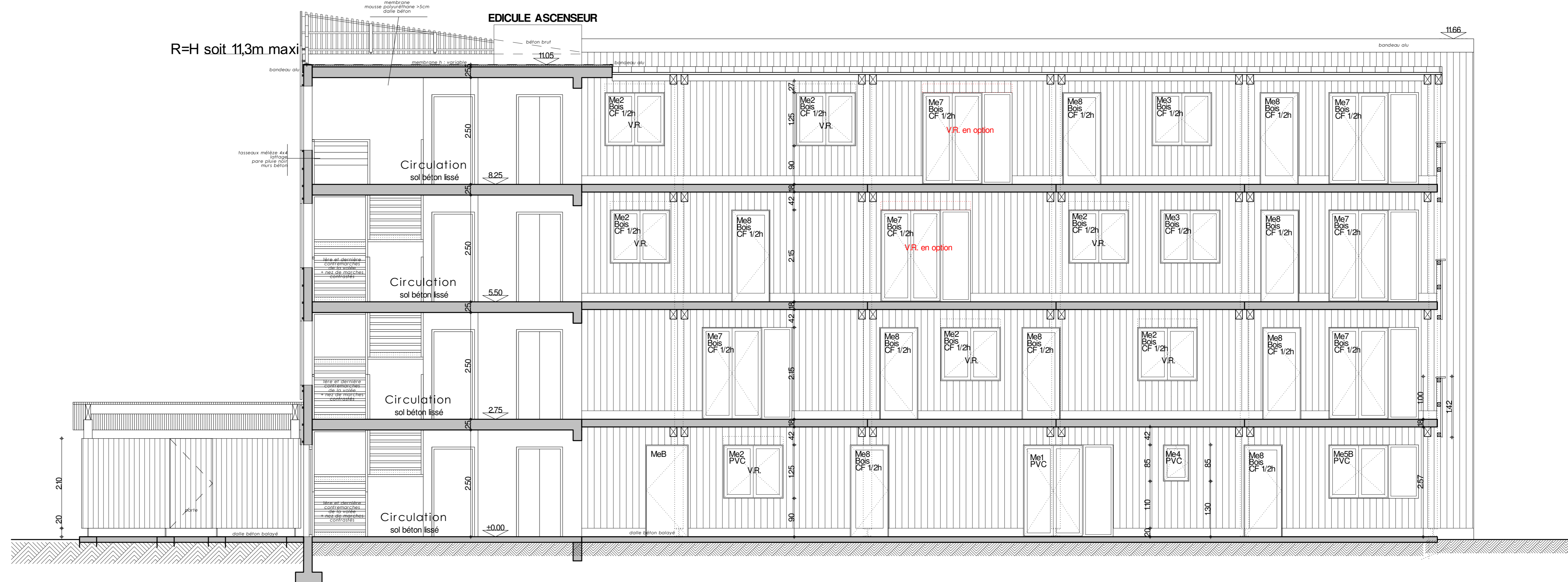
COUPE B - CIRCULATION & COURSIVE
