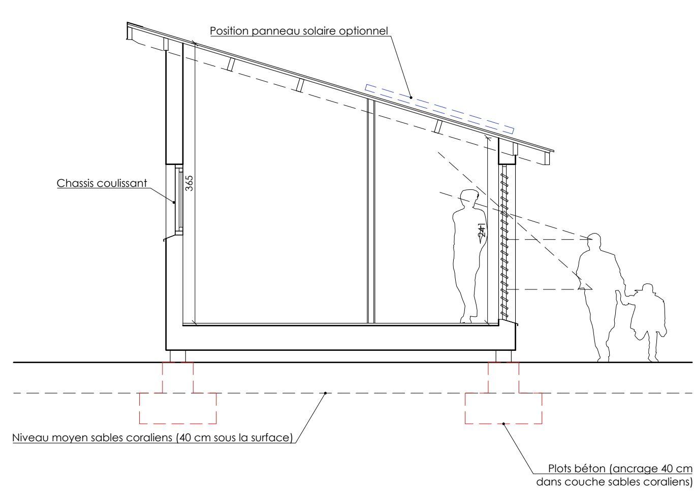
COUPE AA HLL SIMPLE BASE MIROIR CLIMATISE
