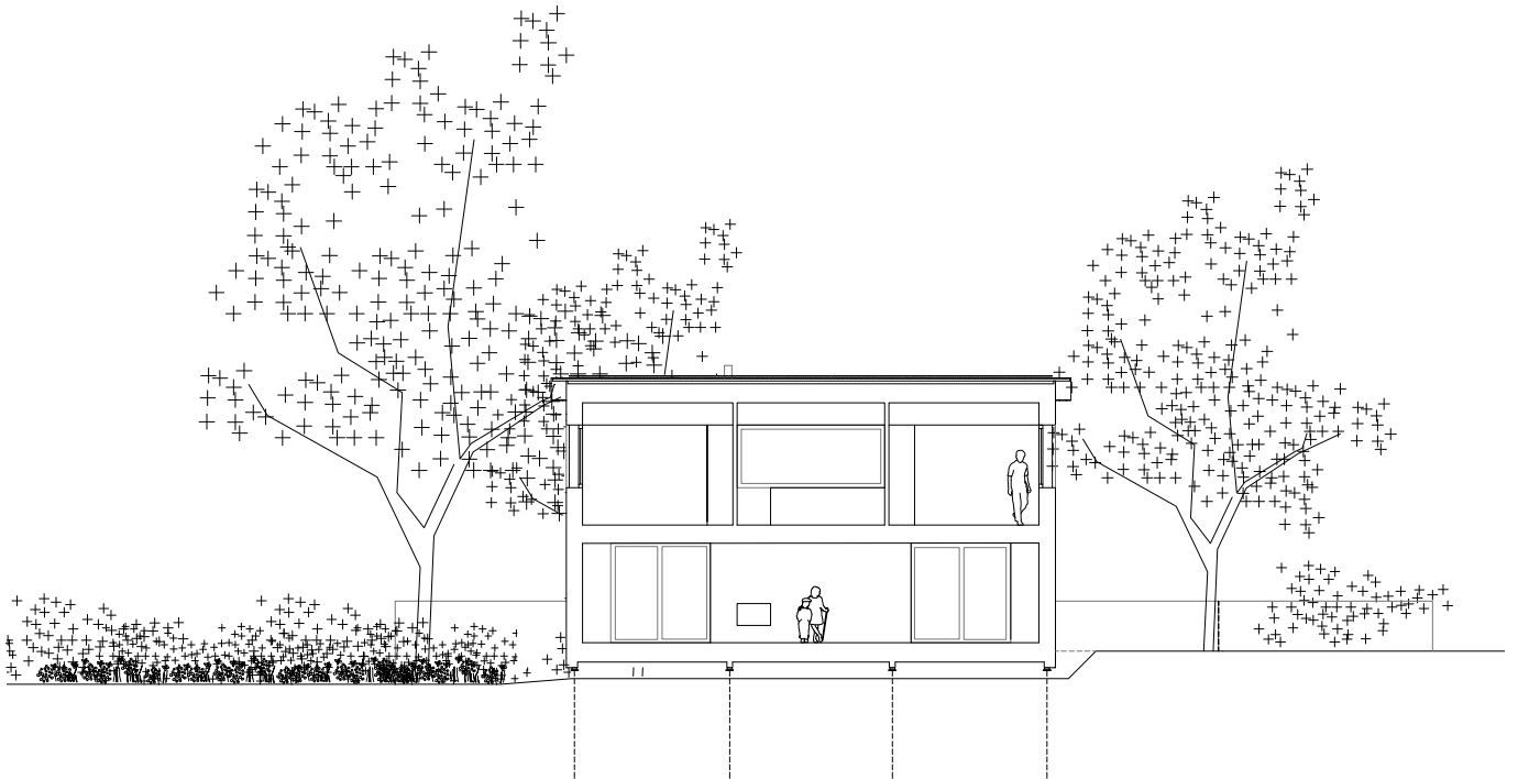
coupe longitudinale - 1:200
