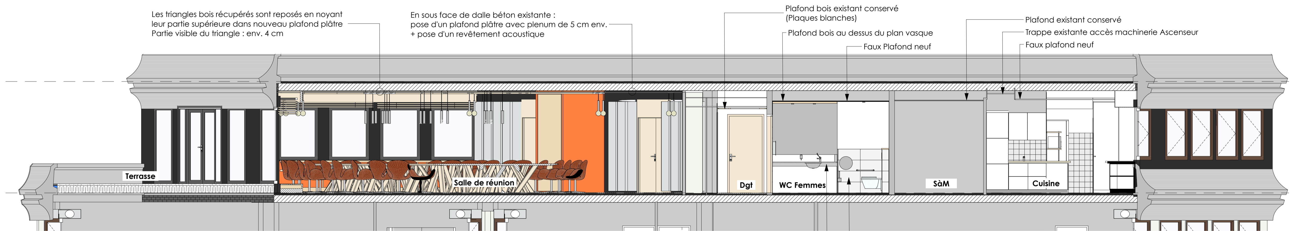
Coupe Longitudinale de principe L1 Echelle : 1/50ème
