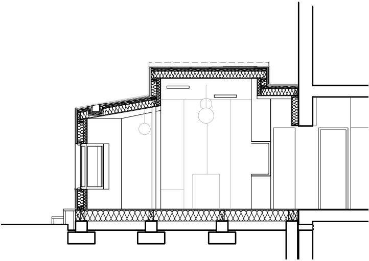
COUPE TRANSVERSALE
