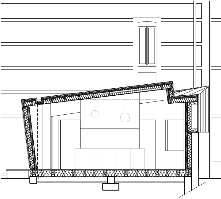
COUPE LONGITUDINALE
