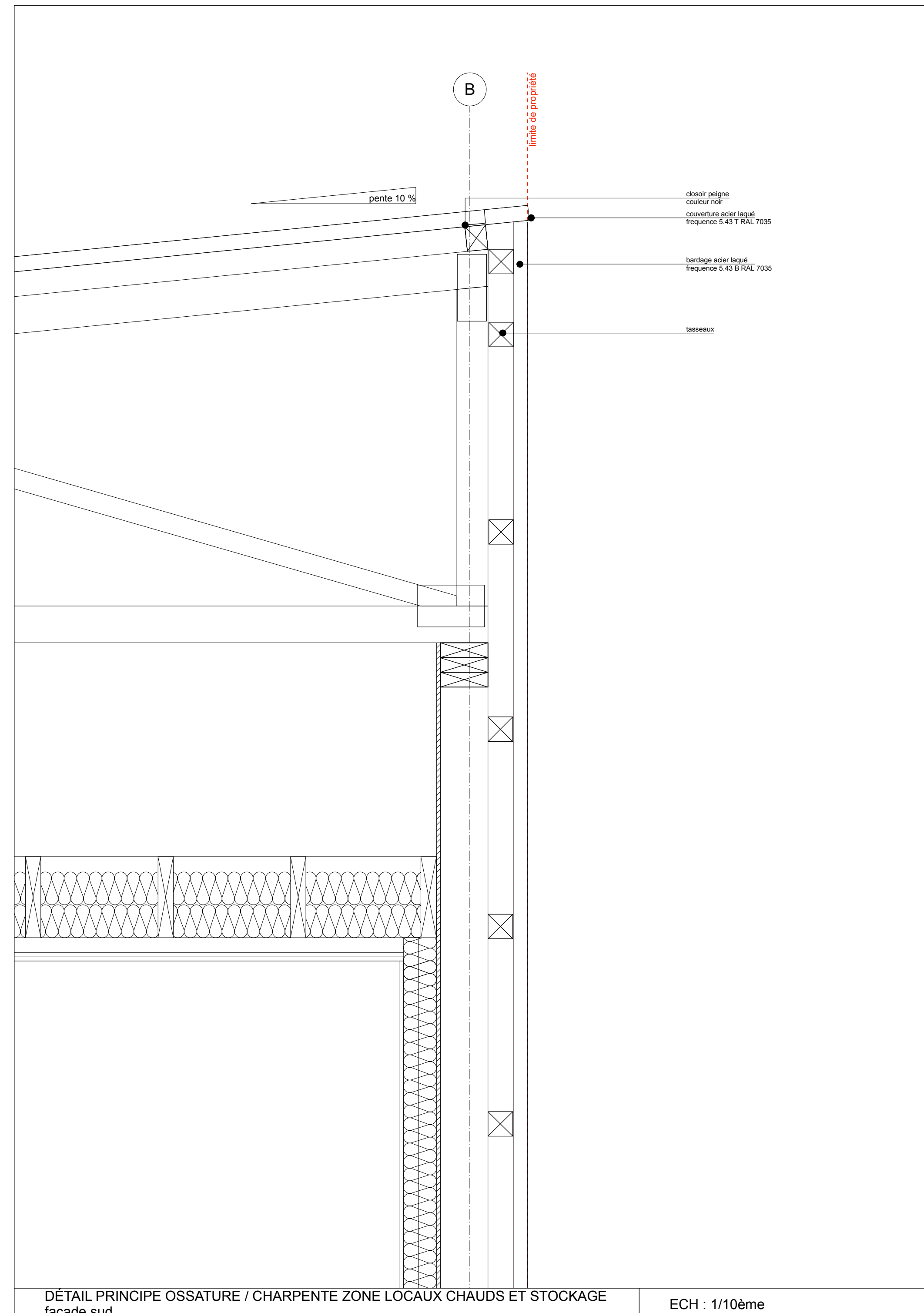
DÉTAIL PRINCIPLE OSSATURE / CHARPENTE ZONE LOCAUX CHAUDS ET STOCKAGE façade sud ECH : 1/10ème
