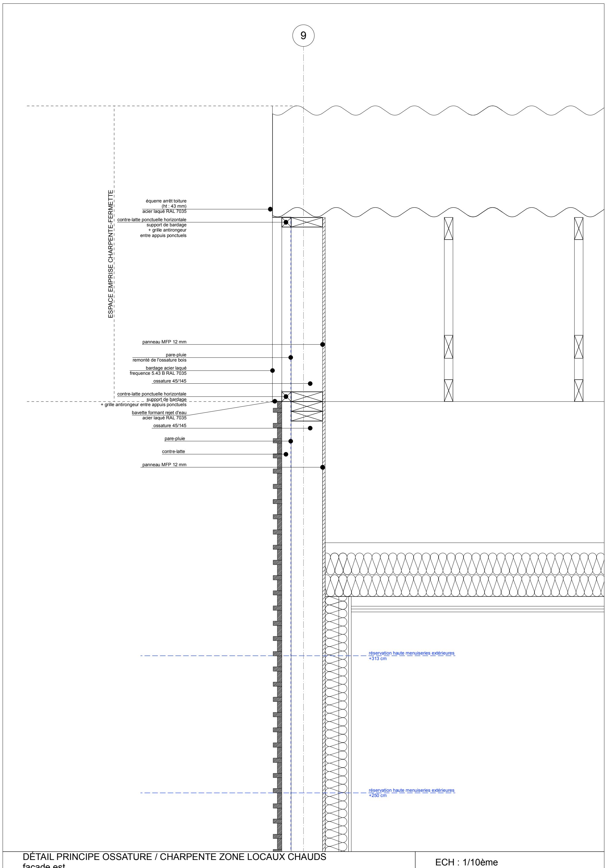
DÉTAIL PRINCIPLE OSSATURE / CHARPENTE ZONE LOCAUX CHAUDS façade est ECH : 1/10ème
