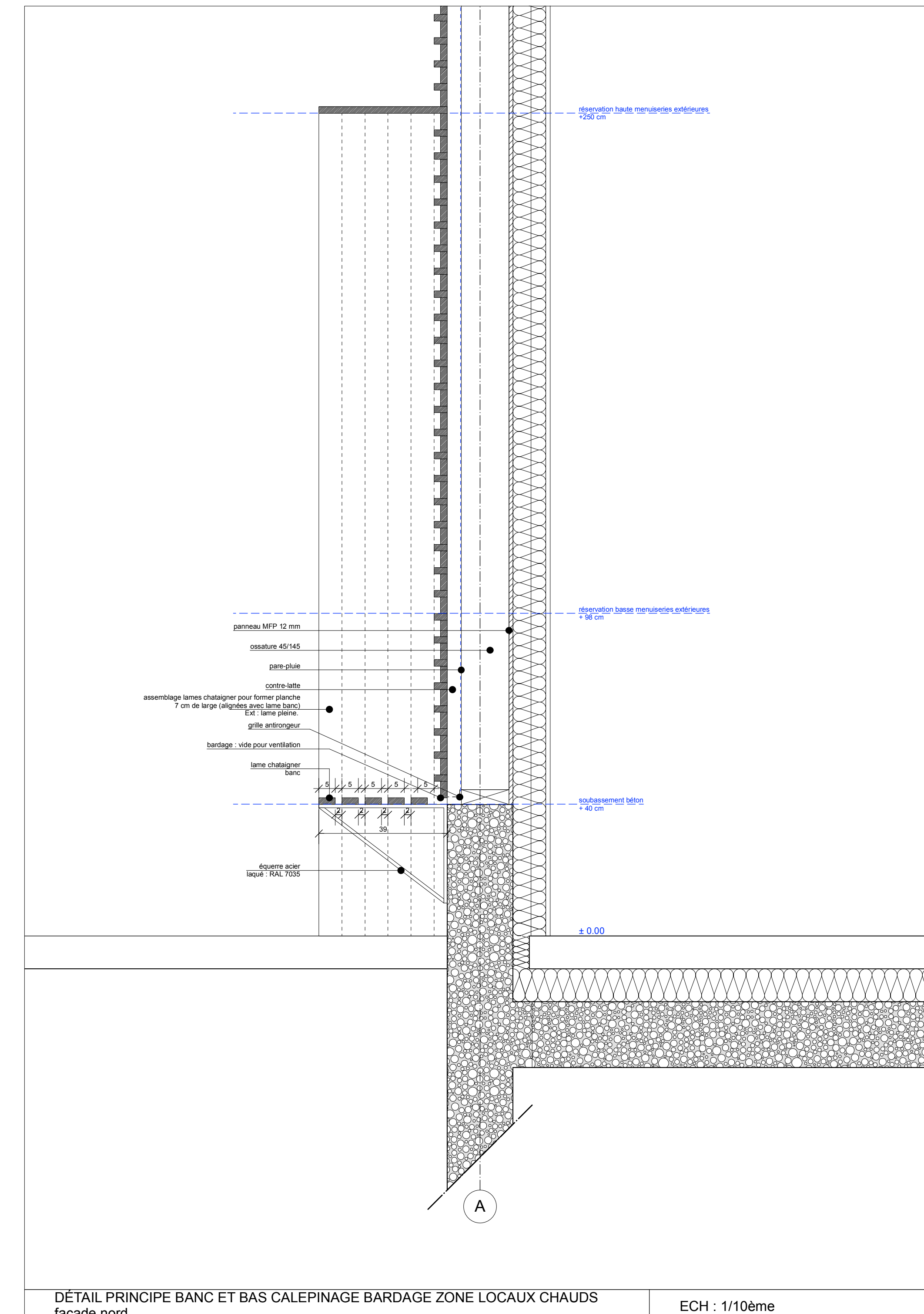
DÉTAIL PRINCIPLE BANC ET BAS CALEPINAGE BARDAGE ZONE LOCAUX CHAUDS façade nord ECH : 1/10ème
