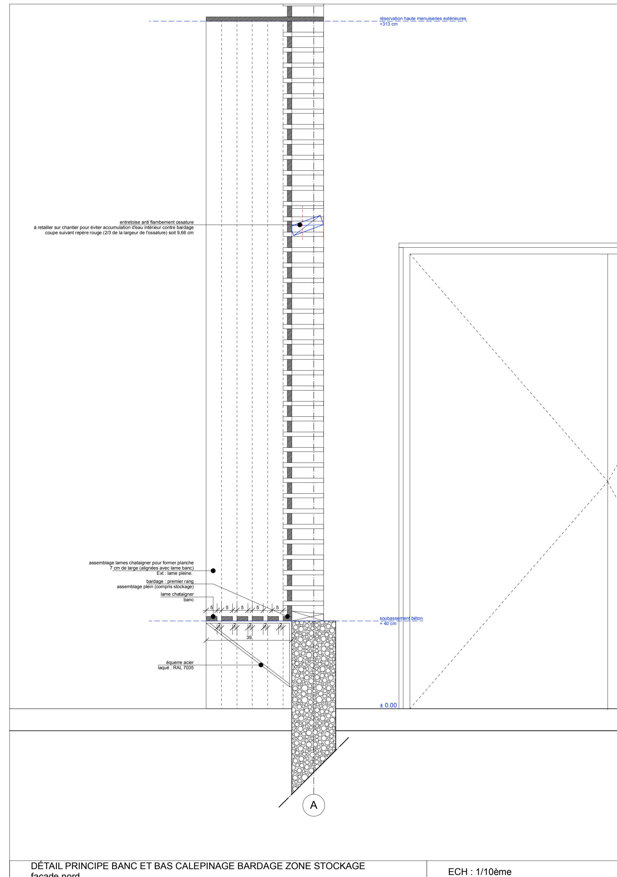
DÉTAIL PRINCIPLE BANC ET BAS CALEPINAGE BARDAGE ZONE STOCKAGE façade nord ECH : 1/10ème
