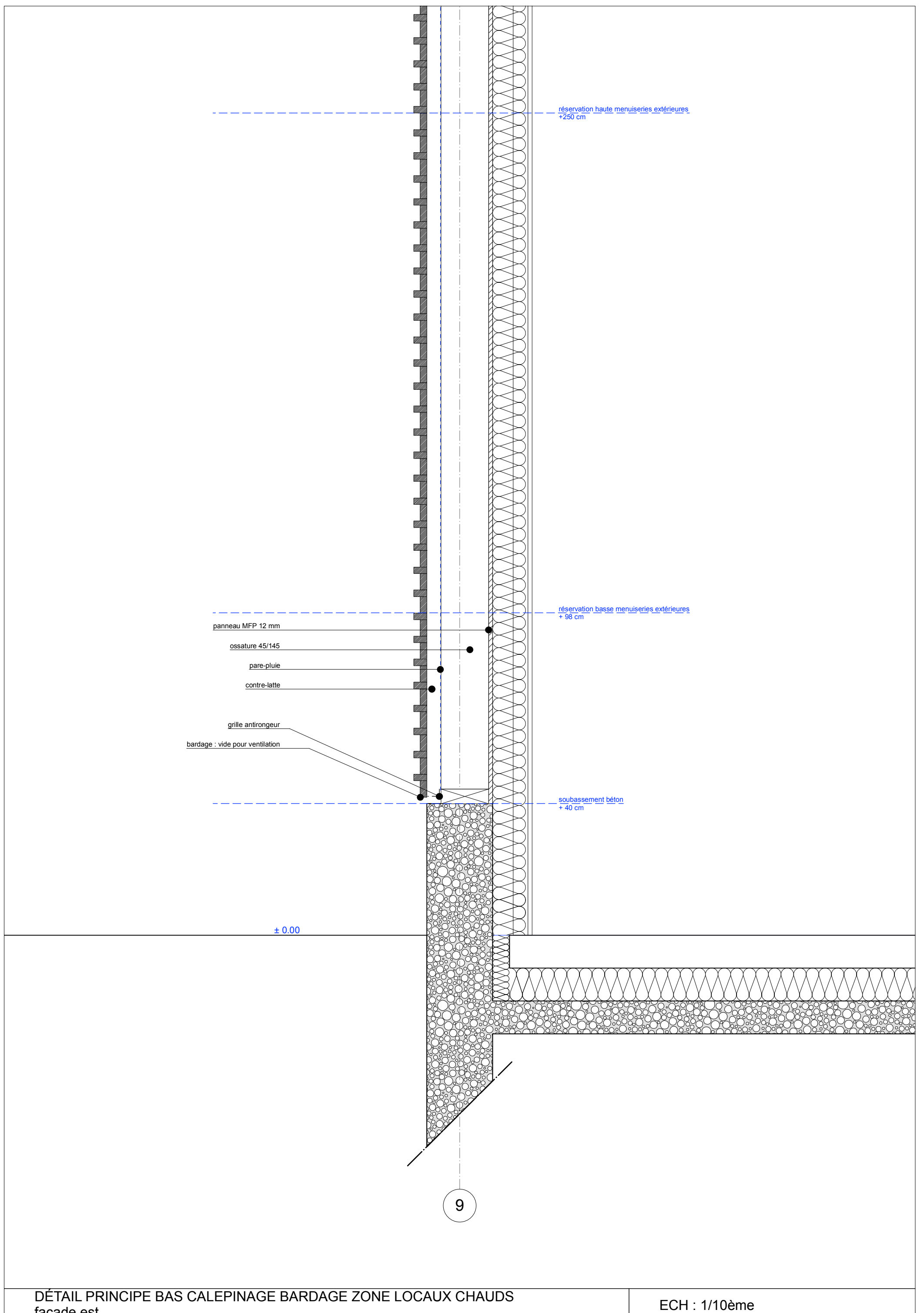
DÉTAIL PRINCIPLE BAS CALEPINAGE BARDAGE ZONE LOCAUX CHAUDS façade est ECH : 1/10ème
