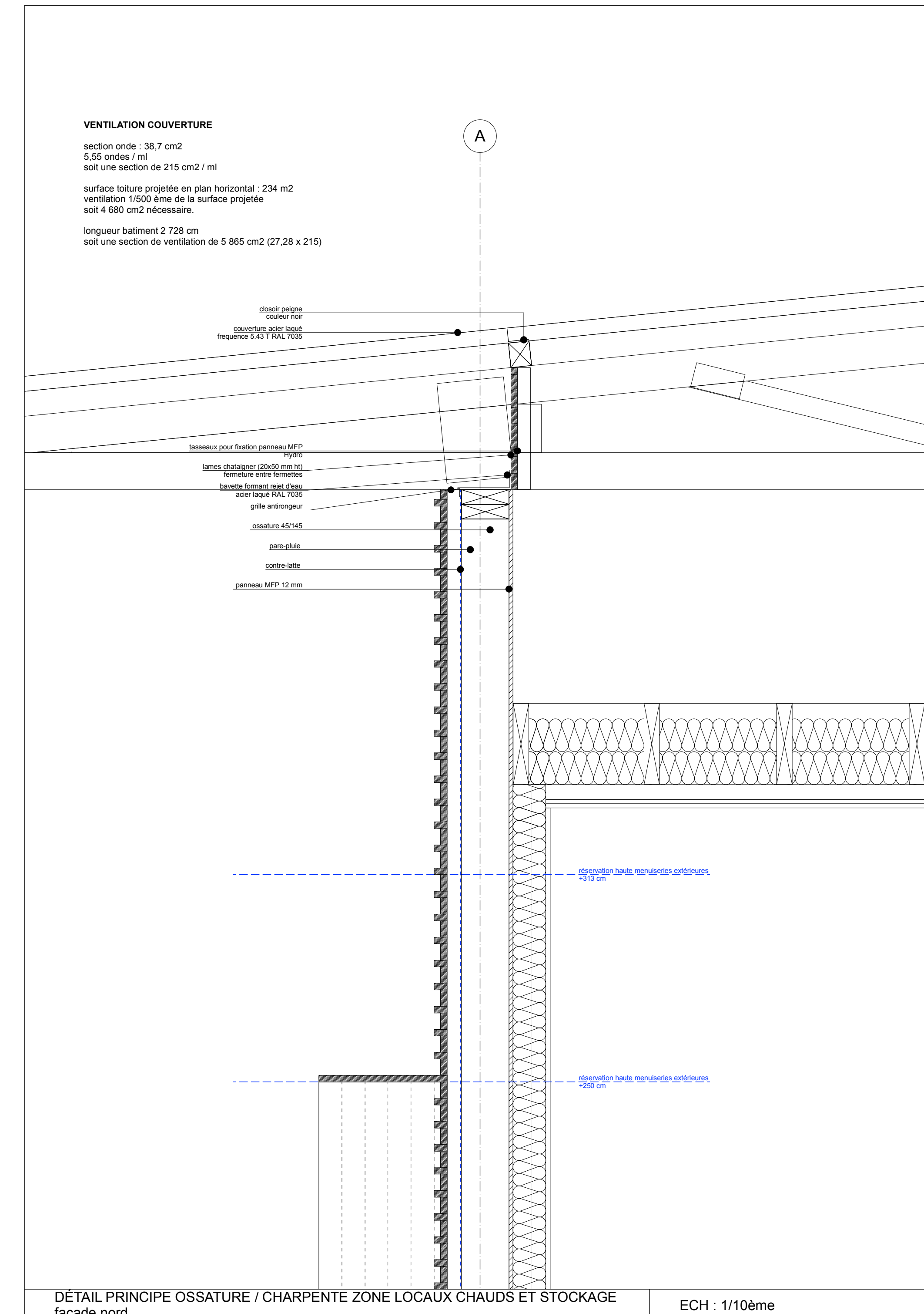
DÉTAIL PRINCIPLE OSSATURE / CHARPENTE ZONE LOCAUX CHAUDS ET STOCKAGE façade nord ECH : 1/10ème
