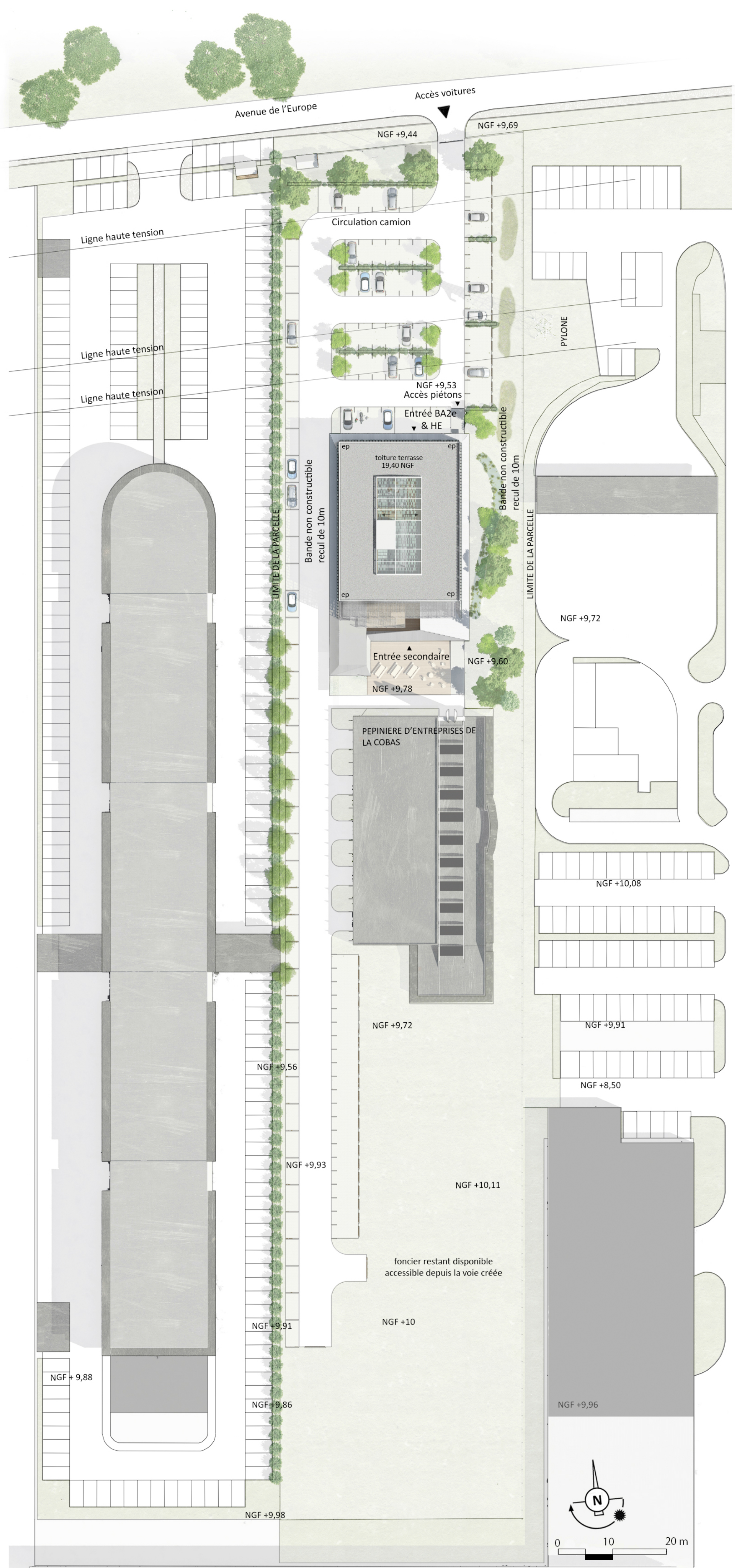
Plan masse - 1/500e - Au sud, un espace fédérateur extérieur est créé entre la pépinière, le siège BA2e et l'hôtel d'entreprises.
